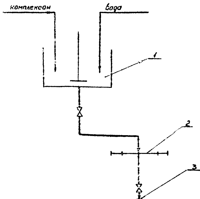
Рис. 1. Схема установки для приготовления и дозирования растворов ингибитора накипесобразования: 1 - реактор растворитель РЗРП-6/250 (сталь Х18НЮТ или Х17Н13М2Т); 2 - мерник МВ-6/25 (сталь Х18НЮТ или Х17Н13М2Т); 3 - точка ввода раствора комплексона.
