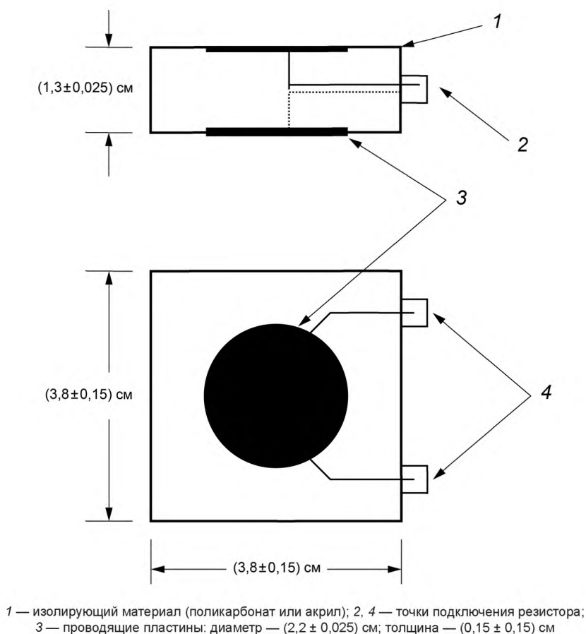
Рисунок 2 — Плоскопараллельный емкостный пробник
