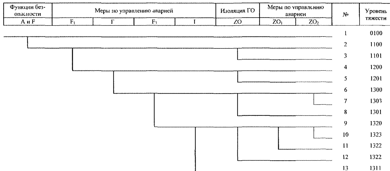
Рисунок 4. Обобщенное дерево событий для аварии с малым и очень малым нарушением целостности границы первого контура
