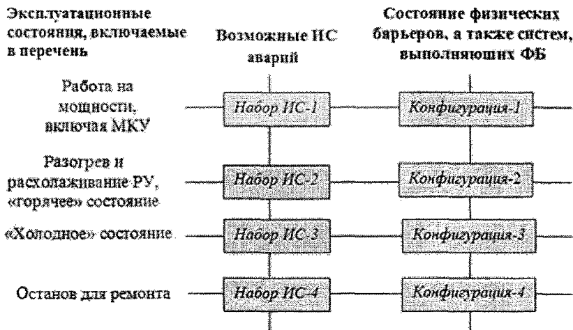
Рисунок 1. Пример составления перечня эксплуатационных состояний АС для реакторной установки в зависимости от возможных ИС аварий, а также состояния физических барьеров и систем АС, выполняющих ФБ
