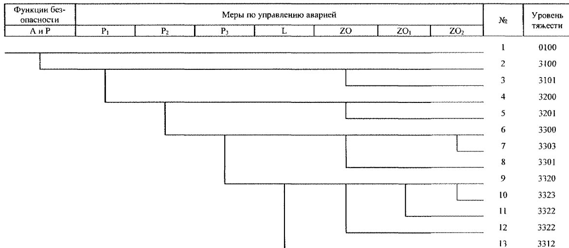
Рисунок 3. Обобщенное дерево событий для аварии без нарушения целостности границы первого контура
