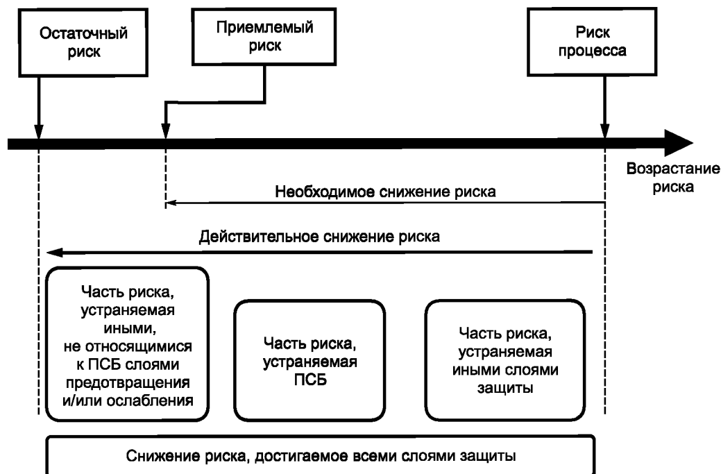
Рисунок А.1 — Общая концепция снижения риска
