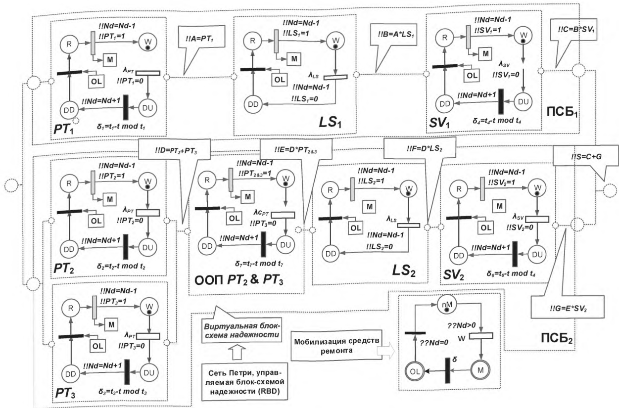
Рисунок J.10 — Моделирование привлечения ресурса ремонта
