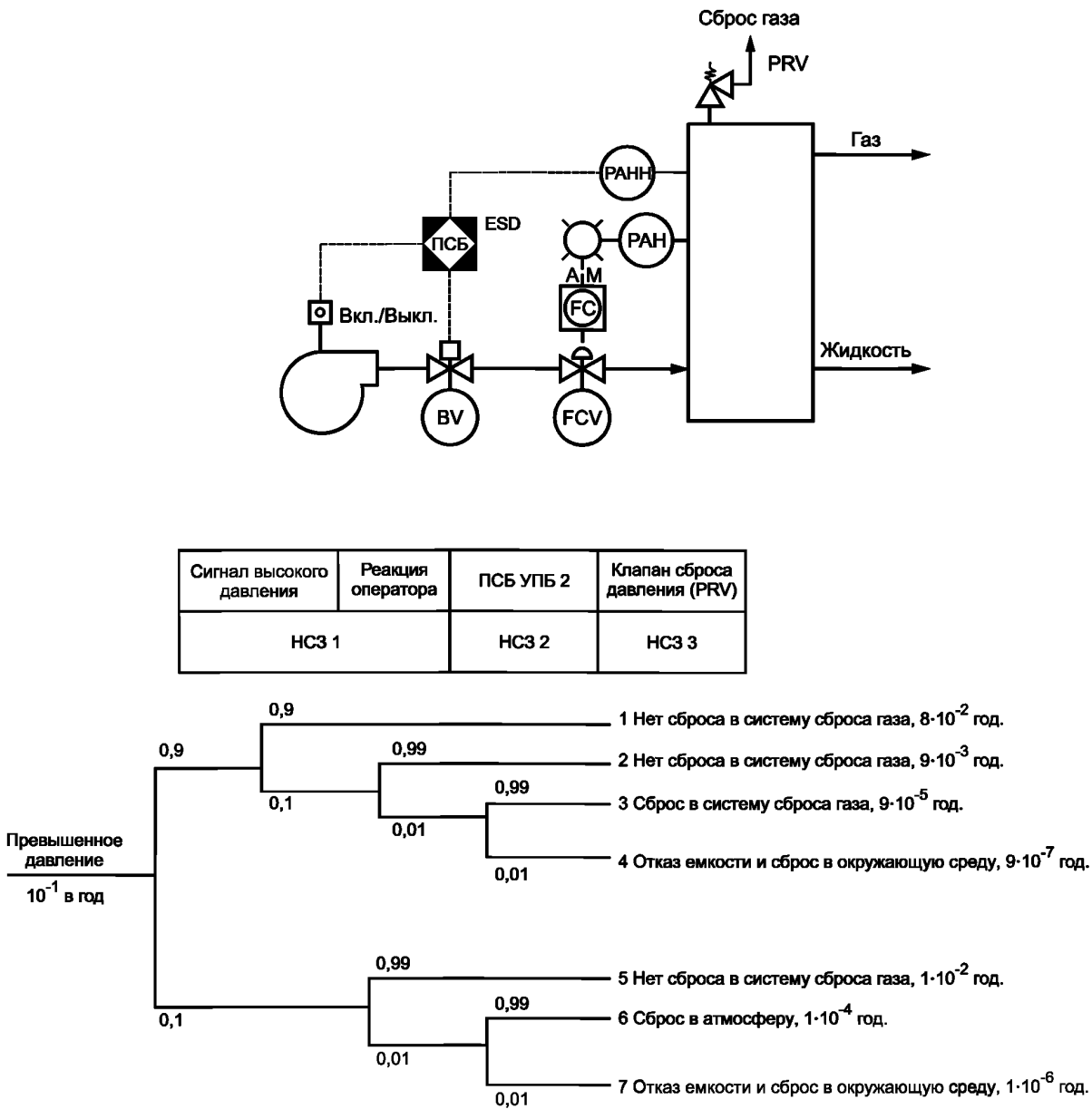
Примечание — Результаты были округлены до первой значащей цифры. Рисунок В.4 — Опасные события для функции безопасности ПСБ с УПБ 2
