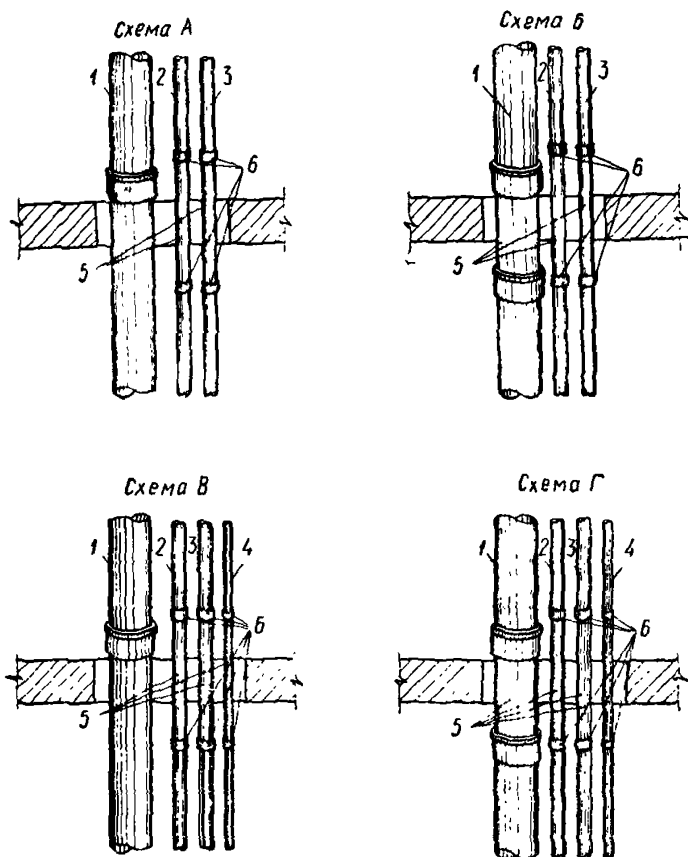
Рис. 6. Схемы соединения стояков санитарно-технических кабин.
