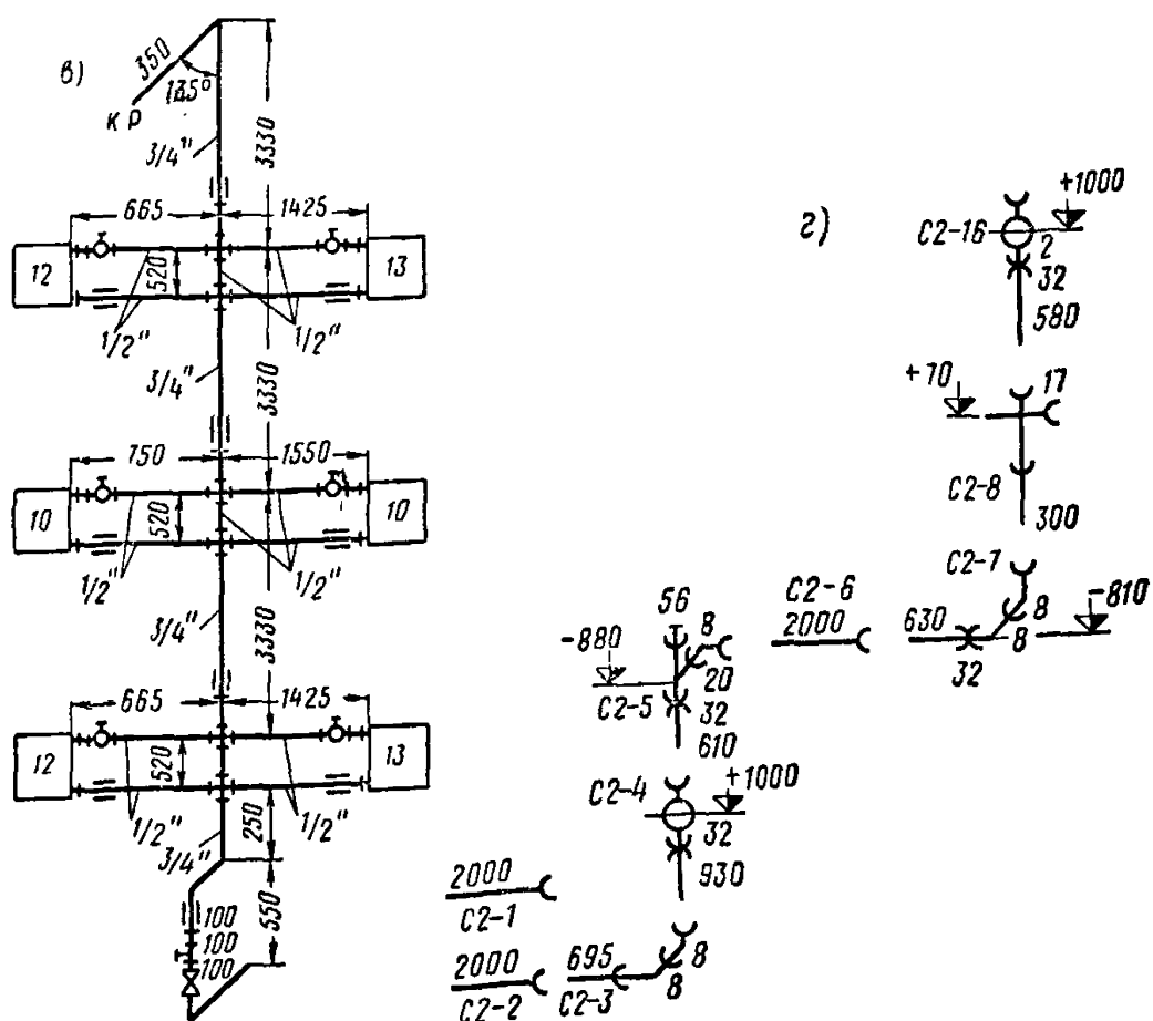
Рис. 1. Замерные эскизы.
