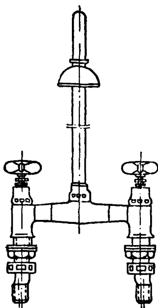
Рис. 22. Настольный смеситель, устанавливаемый на полочку умывальника.
