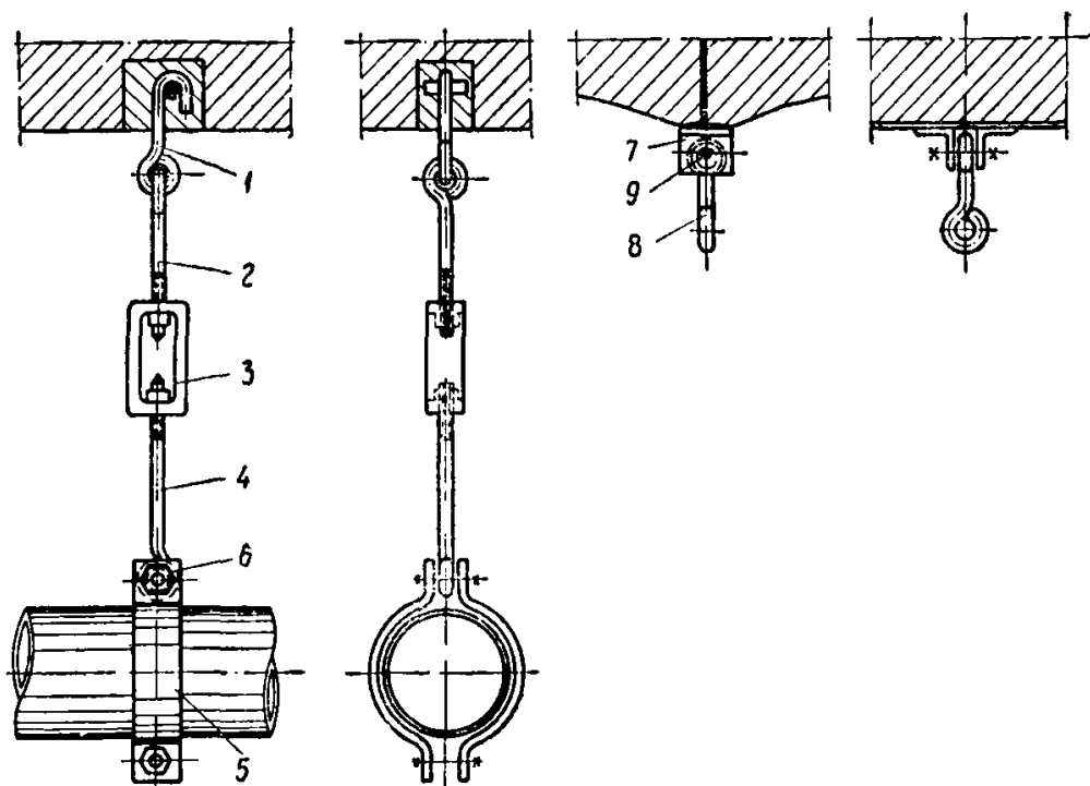
Рис. 27. Подвесная опора.
