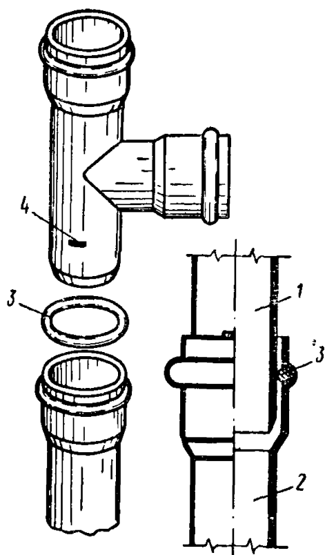
Рис. 2. Раструбные соединения труб и фасонных частей.
