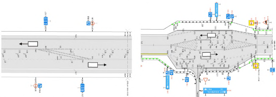
Рисунок - 4.2. Выполнение записи пространственного расположения оси дороги для трёхполосных дорог и в зоне перекрёстков
