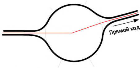
Рисунок - 4.6. Трассирование осевой линии на кольцевой развязке
