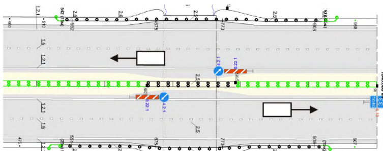
Рисунок - 4.3. Выполнение записи пространственного расположения оси дороги при четырёх и более полосах движения
