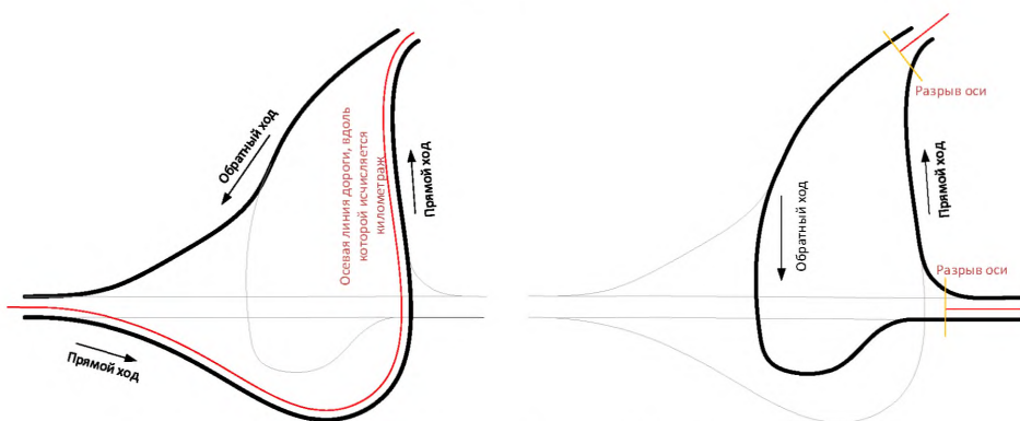
Рисунок - 4.5. Трассирование осевой линии на сложной развязке
