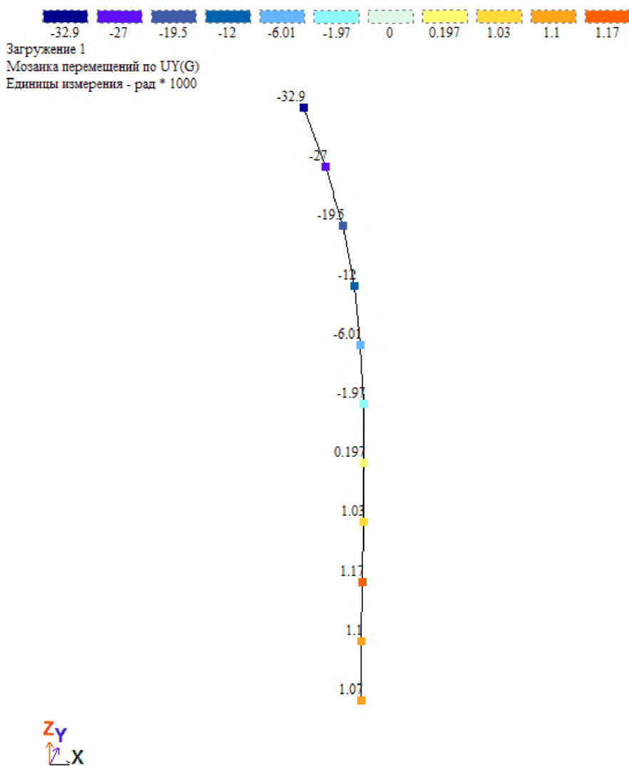
Рисунок В.5 – Мозаики углов поворота точек сваи, рад*1000
