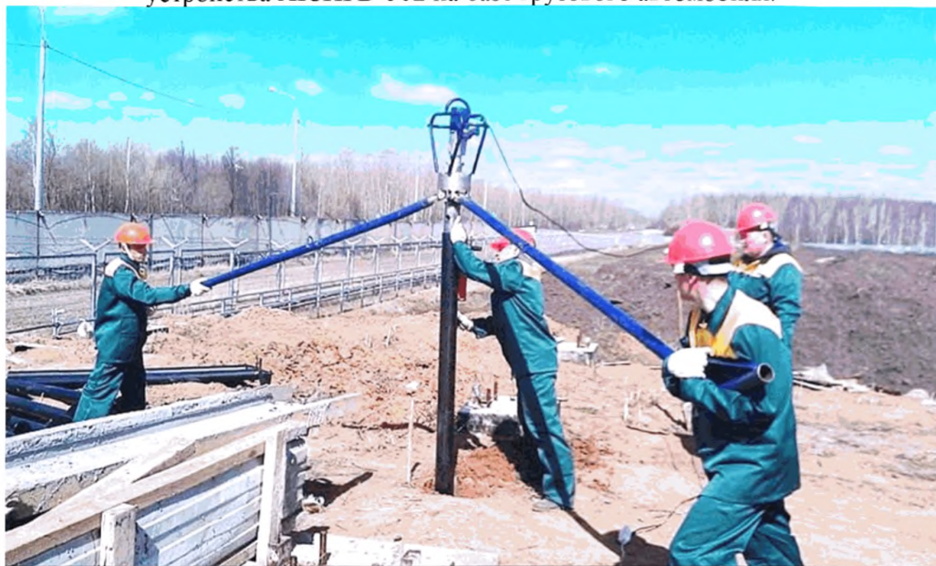
Рисунок Е.1 – Пример монтажа свай СВКС: а) с использованием электрического закручивающего устройства; б) с использованием гидравлического закручивающего устройства AICHI D-502 на базе грузового автомобиля.
