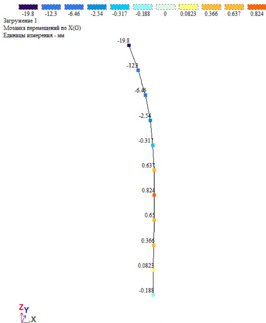
Рисунок В.4 – Мозаика горизонтальных перемещений сваи, мм
