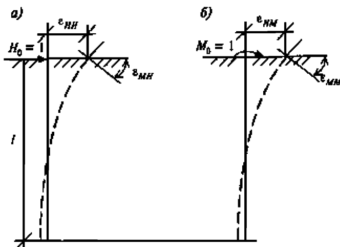
Рисунок В.1 – Схемы перемещения свай в грунте; а) от воздействия горизонтальной силы, б) от воздействия изгибающего момента
