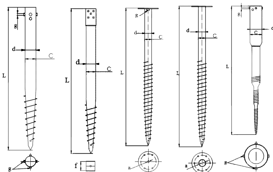
Рисунок А.3 – Примеры разновидностей СВКС
