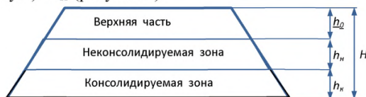
Рисунок 2 – Поперечный профиль насыпи из грунта повышенной влажности с выделением неконсолидируемой (пассивной) и консолидируемой (активной) зон
