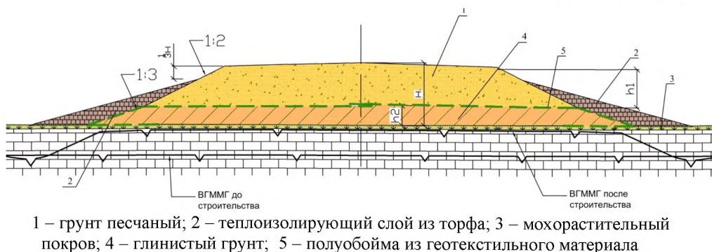
Рисунок 5 – Насыпь переменного профиля из переувлажненного грунта в нижней части
