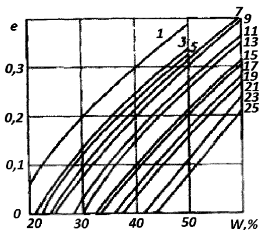
Рисунок 15 – Относительная осадка e песчаных грунтов основания при оттаивании под нагрузкой 0,075 МПа
