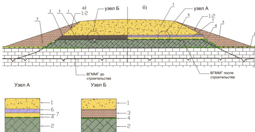
Рисунок 3 – Насыпь из мерзло-комковатого грунта с теплоизолирующими слоями
