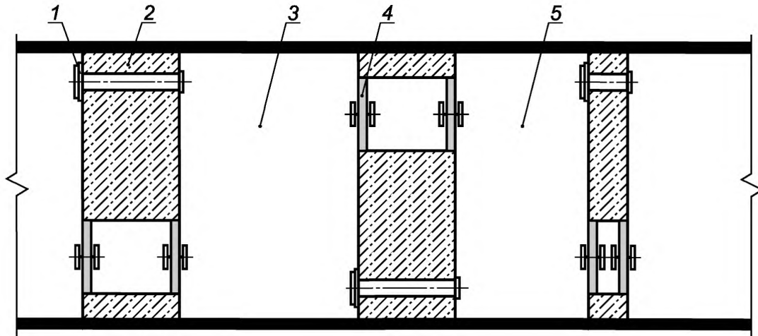
1 — клапан избыточного давления; 2 — взрывоустойчивая перемычка; 3 — тамбур-шлюз; 4 — дверь защитно-герметическая; 5 — шлюзовая камера
