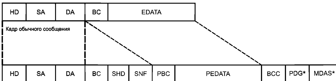
Кадр защищенного сообщения
