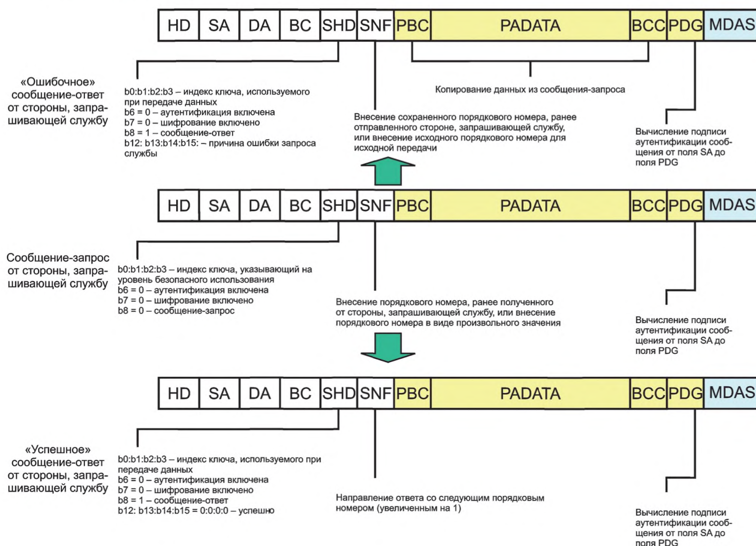
Рисунок 14 — Кадры защищенного сообщения, использующие службу шифрования и службу проверки подлинности данных
