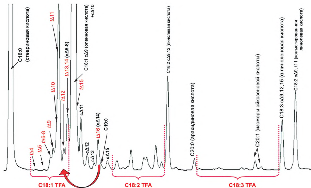
Рисунок В.2 — Пример ГЖХ-хроматограммы молочного продукта [увеличенная область C18:1 ТЖК, C18:2 ТЖК, C18:3 ТЖК и конъюгированная линолевая кислота ( CLA )] с использованием ввода пробы непосредственно в колонку
