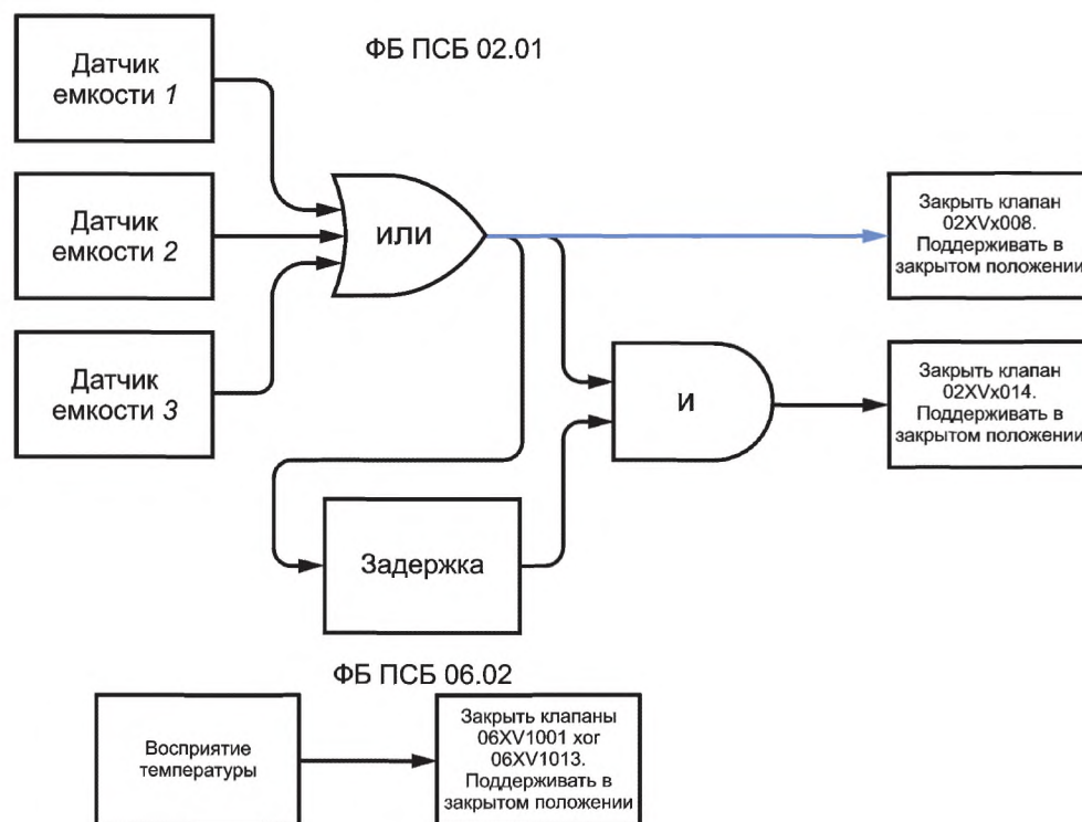
Рисунок В.3 — Функциональная спецификация ФБ ПСБ 02.01 и ФБ ПСБ 06.02
