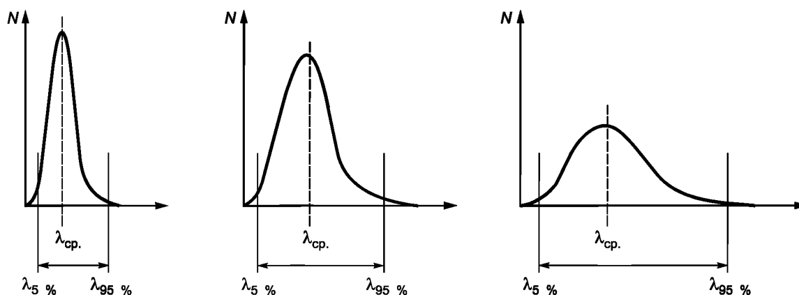
Рисунок A.5 — Иллюстрация погрешности для параметра безотказности
