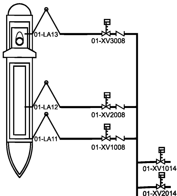
Рисунок В.1 — Технологическая схема для ФБ ПСБ 02.01
