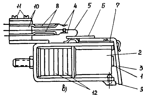
Рис. 8. Общий вид реле серии КДР:
