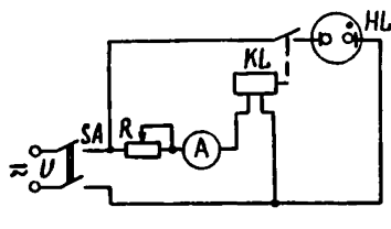
Рис. 17. Схема проверки тока срабатывания и возврата реле
