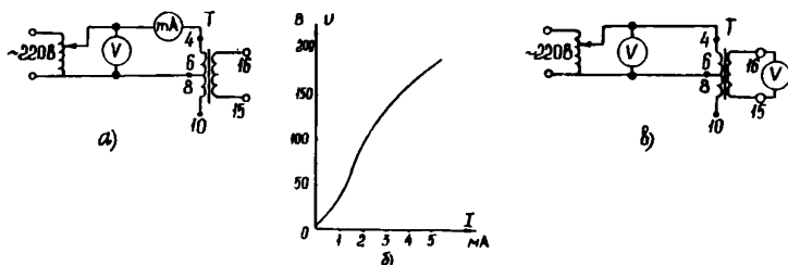
Рис. 27. Схемы проверки трансформатора реле РИC-Э2М, РИC-Э2М-0,2:
