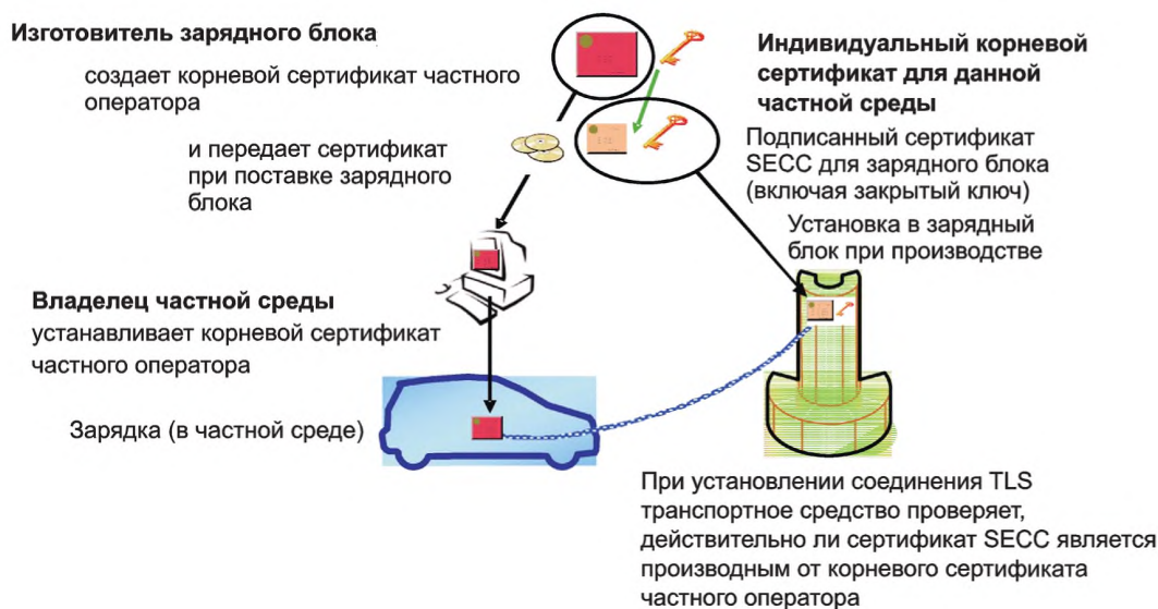
Рисунок С.2 — Зарядка в частной среде
