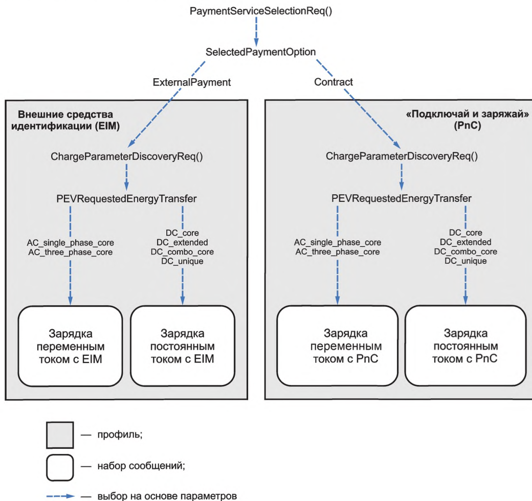
Рисунок 97 — Выбор наборов сообщений
