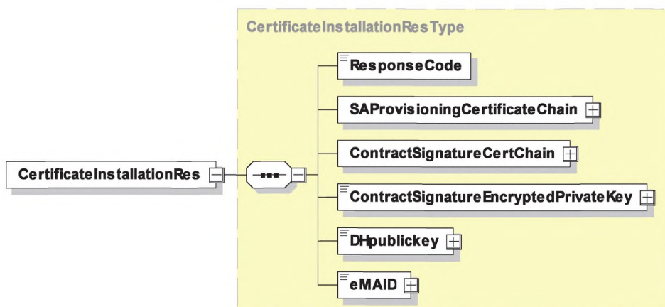
Рисунок 42 — Диаграмма — CertificateInstallationRes
