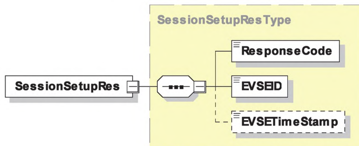
Рисунок 24 — Диаграмма — SessionSetupRes
