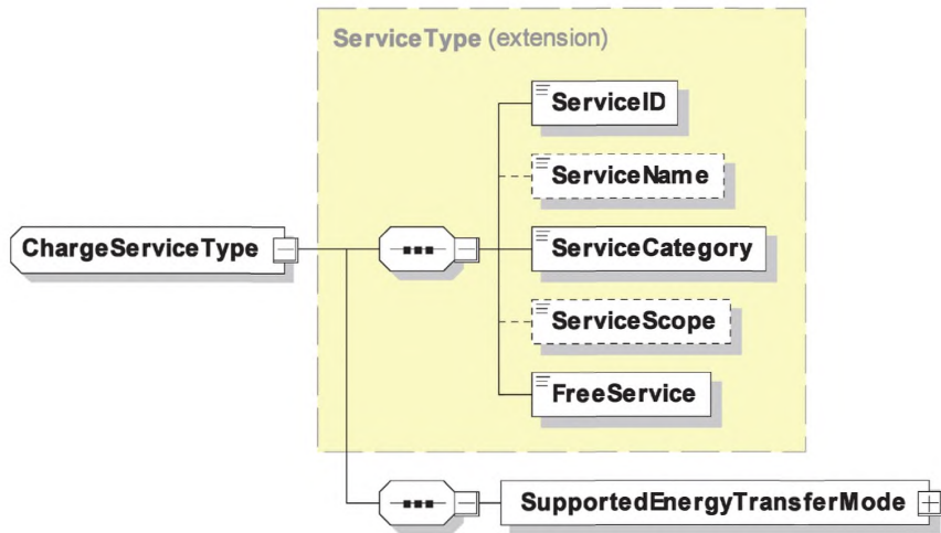
Рисунок 59 — Диаграмма — ChargeServiceType
