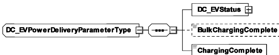
Рисунок 94 — Диаграмма — DC_EVPowerDeliveryParameterType
