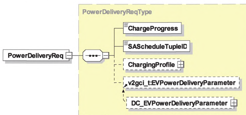
Рисунок 37 — Диаграмма — PowerDeliveryReq
