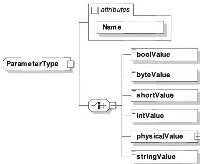
Рисунок 79 — Диаграмма — ParameterType
