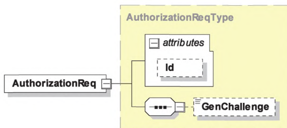
Рисунок 33 — Диаграмма — AuthorizationReq
