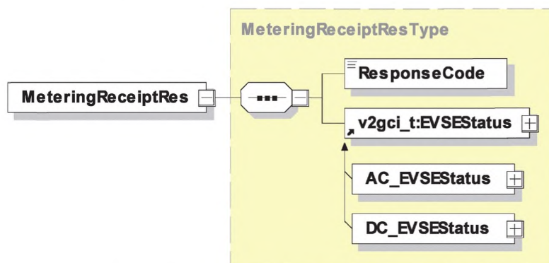
Рисунок 46 — Диаграмма — MeteringReceiptRes
