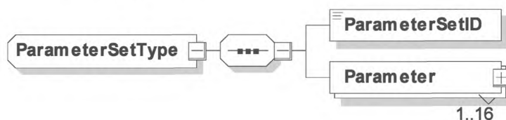
Рисунок 78 — Диаграмма — ParameterSetType
