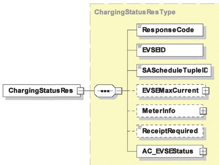
Рисунок 48 — Диаграмма — ChargingStatusRes
