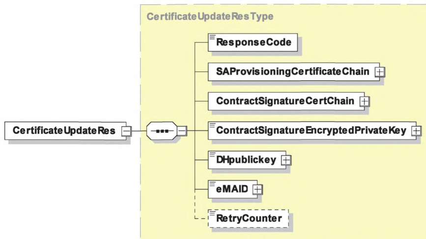
Рисунок 40 — Диаграмма — CertificateUpdateRes
