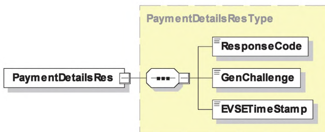
Рисунок 32 — Диаграмма — PaymentDetailsRes
