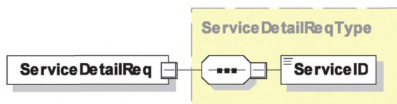
Рисунок 27 — Диаграмма — ServiceDetailReq
