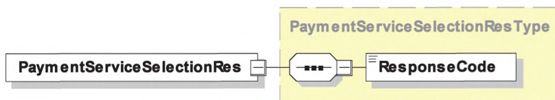
Рисунок 30 — Диаграмма — PaymentServiceSelectionRes
