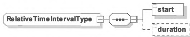
Рисунок 74 — Диаграмма — RelativeTimeIntervalType
