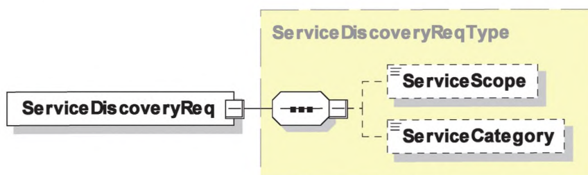
Рисунок 25 — Диаграмма — ServiceDiscoveryReq
