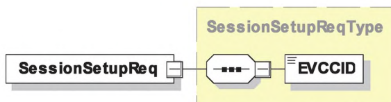
Рисунок 23 — Диаграмма — SessionSetupReq
