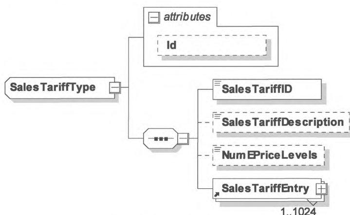
Рисунок 72 — Диаграмма — SalesTariffType
