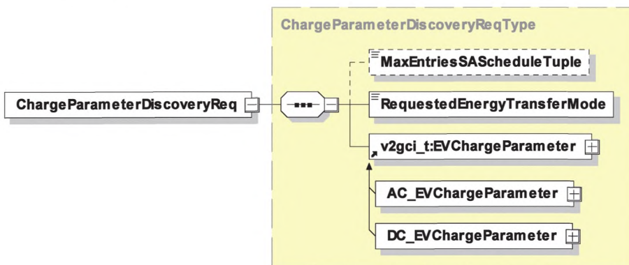
Рисунок 35 — Диаграмма — ChargeParameterDiscoveryReq
