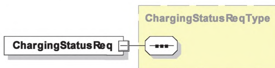
Рисунок 47 — Диаграмма — ChargingStatusReq
