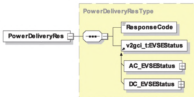
Рисунок 38 — Диаграмма — PowerDeliveryRes
