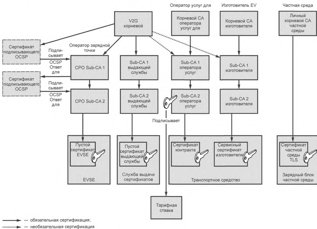
Рисунок С.1 — Обзор структуры сертификатов
