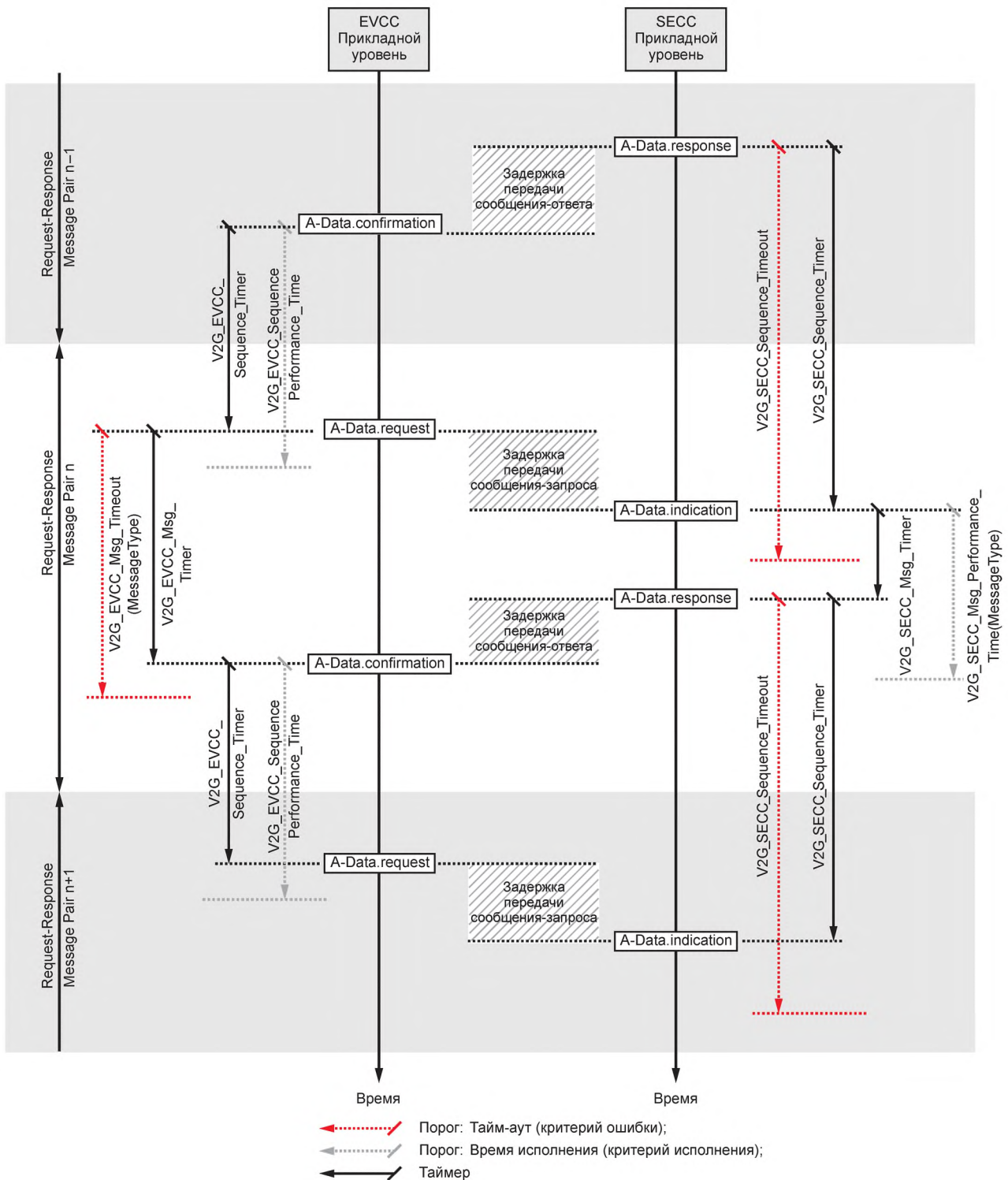
Рисунок 98 — Хронирование последовательности сообщений и сеанса связи
