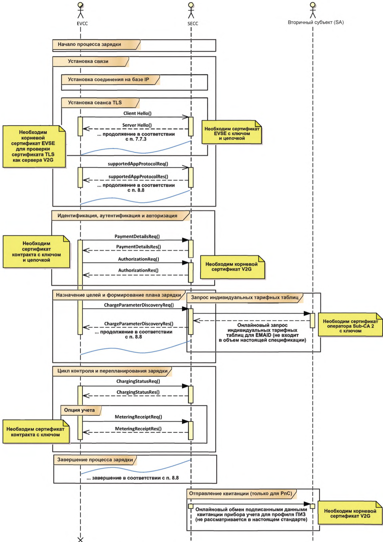
Рисунок 5 — Пример связи в онлайн-режиме
