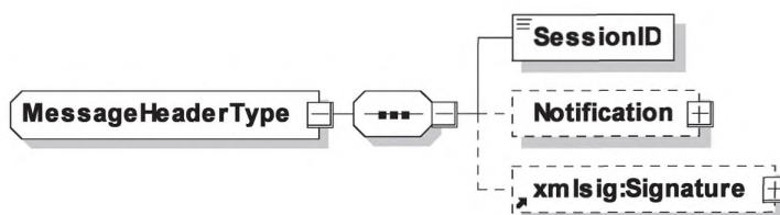
Рисунок 20 — Диаграмма — Заголовок сообщения
