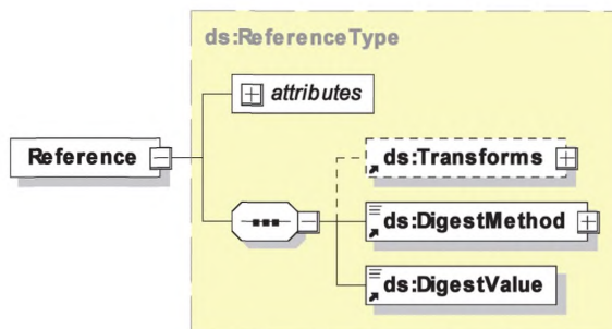
Рисунок 13 — Диаграмма — Элемент Reference, включенный в элемент SignedInfo
