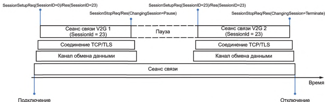
Рисунок 22 — Обработка сеанса связи V2G
