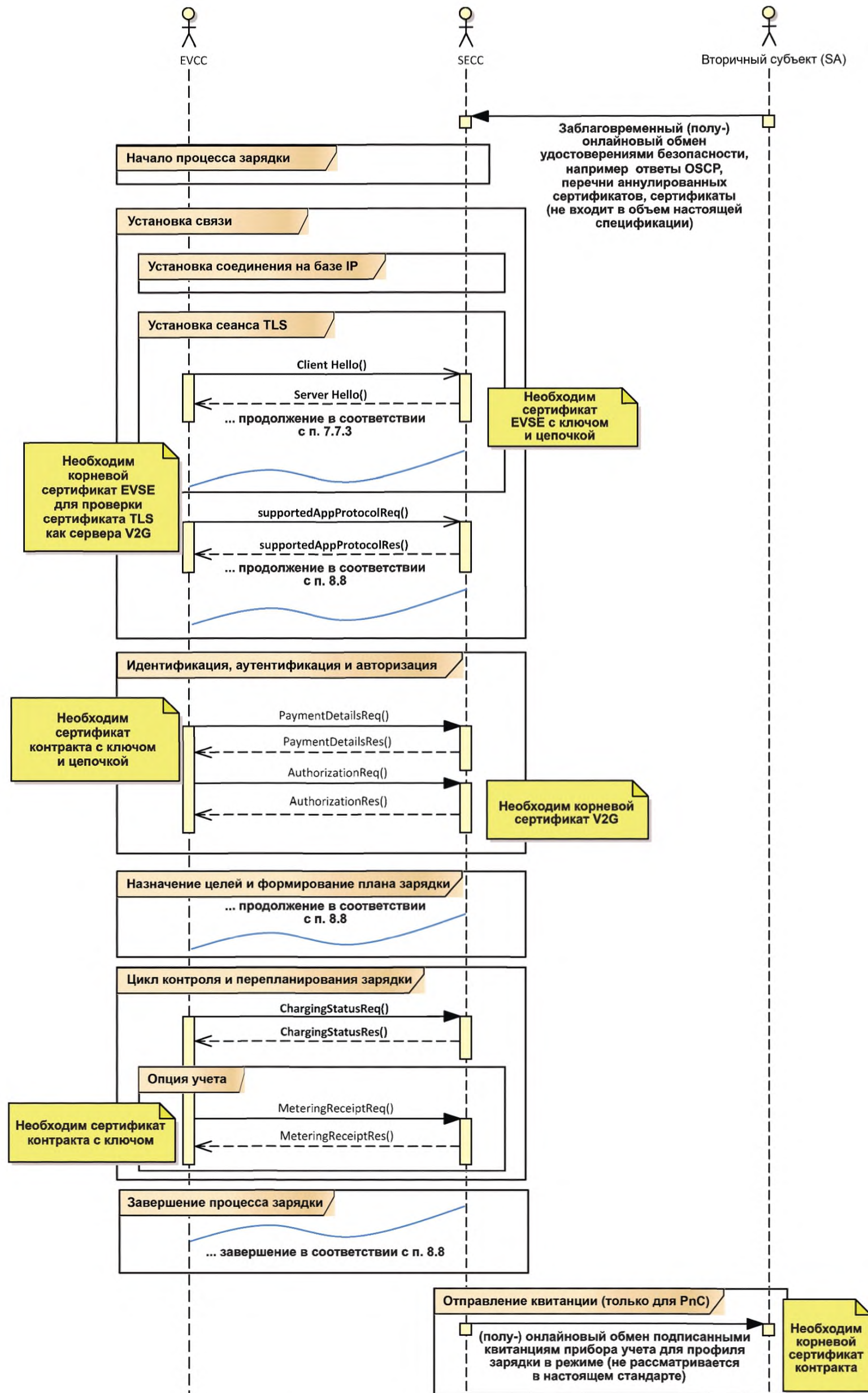
Рисунок 4 — Пример связи в полуонлайн режиме
