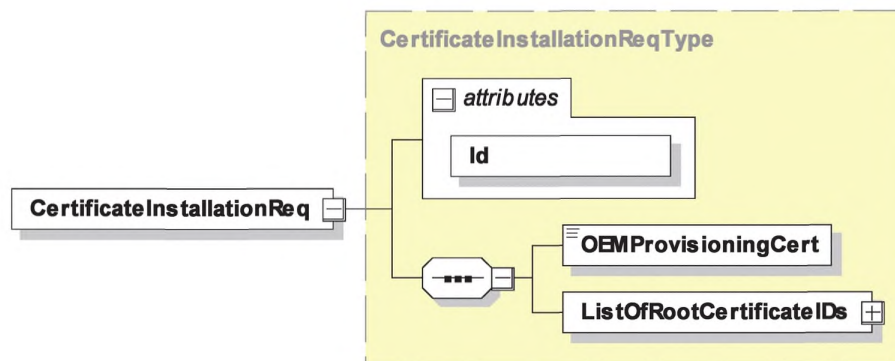
Рисунок 41 — Диаграмма — CertificateInstallationReq
