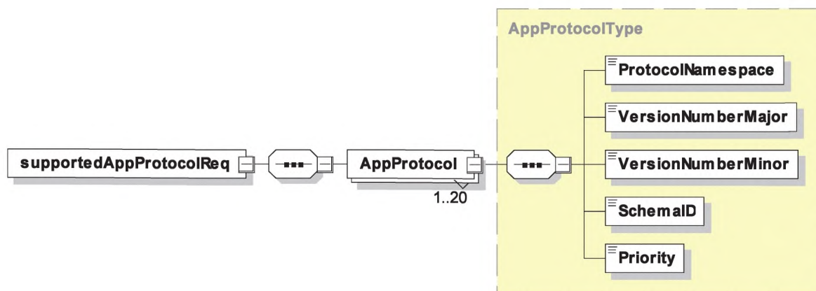
Рисунок 17 — Диаграмма — supportedAppProtocolReq
