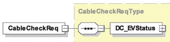
Рисунок 49 — Диаграмма — CableCheckReq
