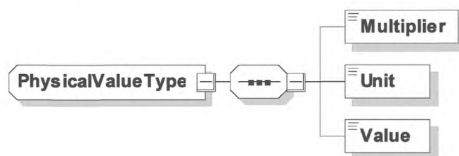
Рисунок 63 — Диаграмма — PhysicalValueType
