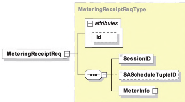
Рисунок 45 — Диаграмма — MeteringReceiptReq
