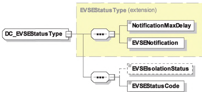
Рисунок 90 — Диаграмма — DC_EVSEStatusType
