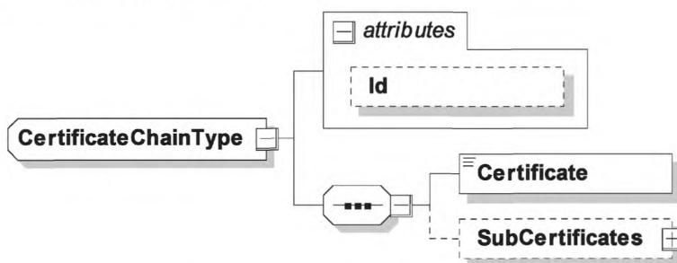
Рисунок 61 — Диаграмма — CertificateChainType
