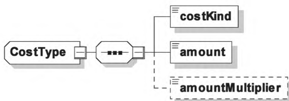
Рисунок 76 — Диаграмма — CostType
