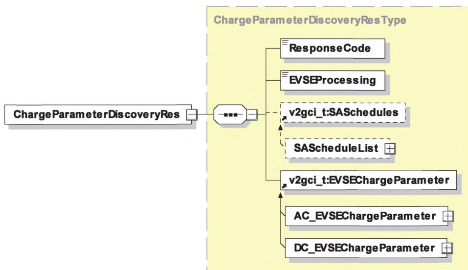
Рисунок 36 — Диаграмма — ChargeParameterDiscoveryRes
