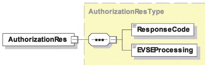
Рисунок 34 — Диаграмма — AuthorizationRes
