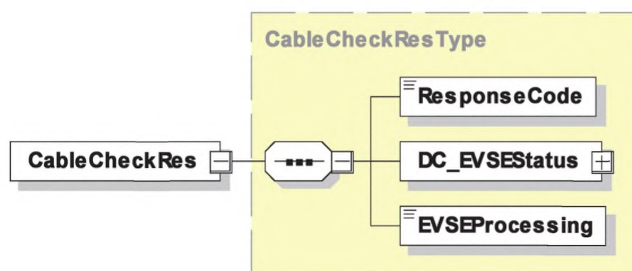
Рисунок 50 — Диаграмма — CableCheckRes
