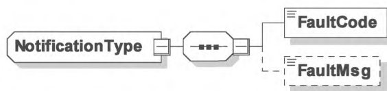
Рисунок 64 — Диаграмма — NotificationType
