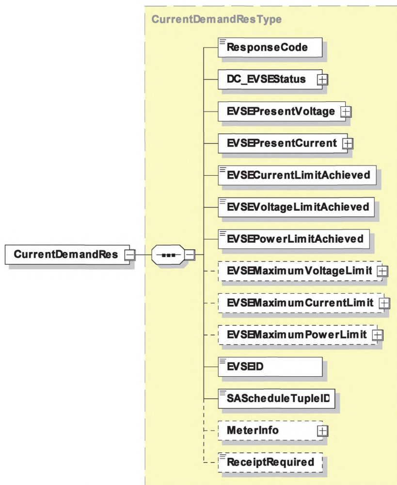
Рисунок 54 — Диаграмма — CurrentDemandRes
