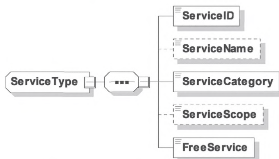
Рисунок 57 — Диаграмма — ServiceType
