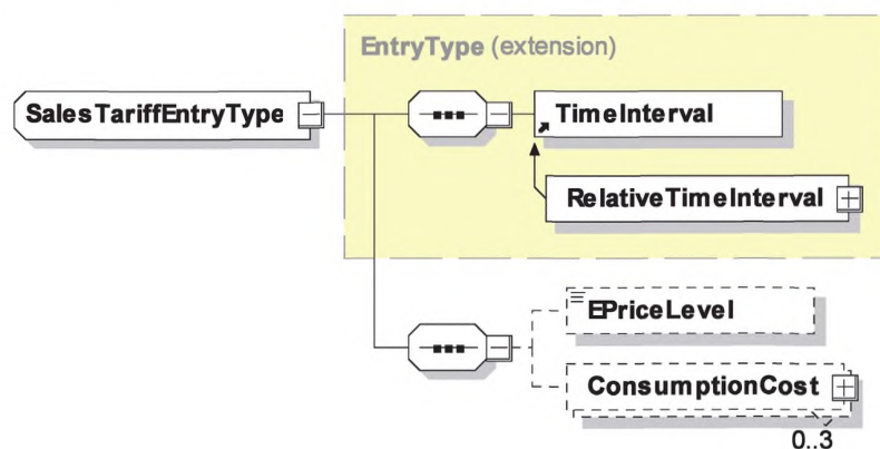
Рисунок 73 — Диаграмма — SalesTariffEntryType
