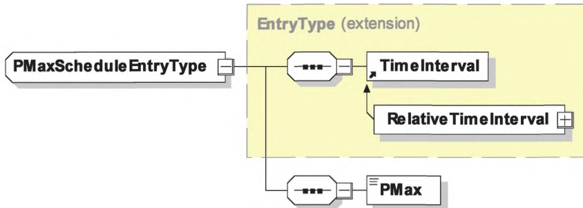
Рисунок 71 — Диаграмма — PMaxScheduleEntryType
