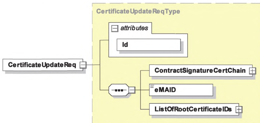
Рисунок 39 — Диаграмма — CertificateUpdateReq
