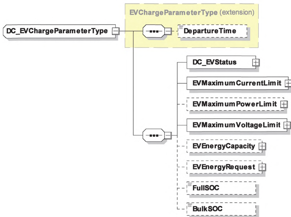
Рисунок 92 — Диаграмма — DC_EVChargeParameterType
