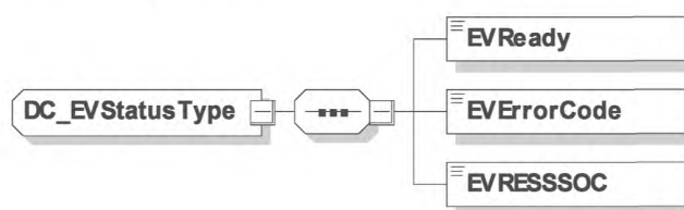
Рисунок 91 — Диаграмма — DC_EVStatusType
