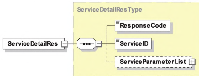
Рисунок 28 — Диаграмма — ServiceDetailRes
