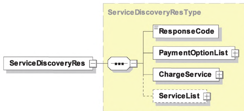
Рисунок 26 — Диаграмма — ServiceDiscoveryRes
