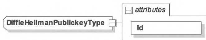
Рисунок 85 — Диаграмма — DiffieHellmanPublicKeyType
