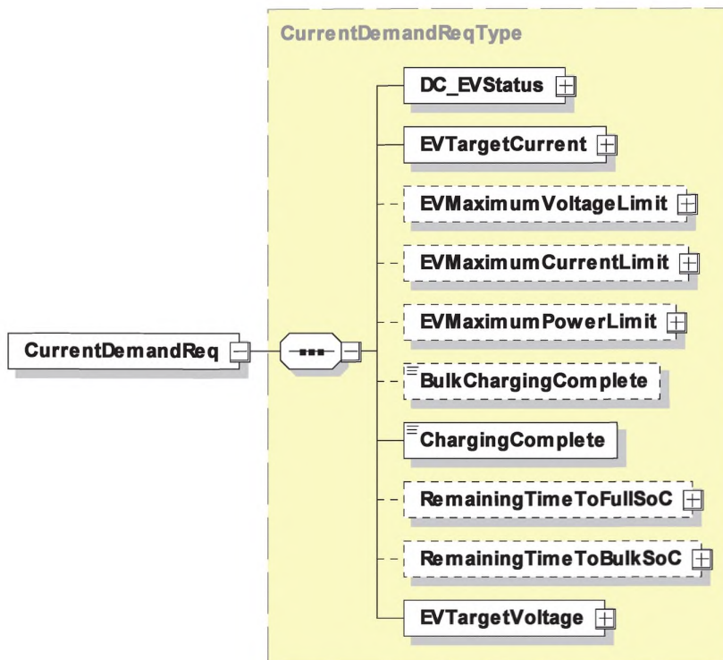
Рисунок 53 — Диаграмма — CurrentDemandReq
