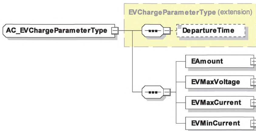
Рисунок 88 — Диаграмма — AC_EVChargeParameterType
