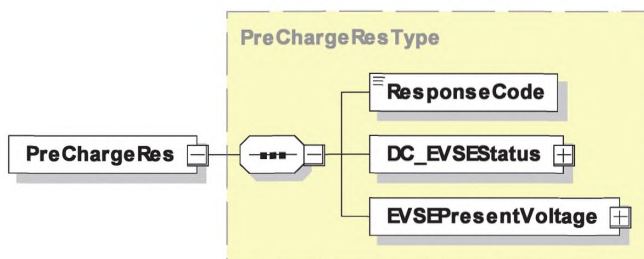
Рисунок 52 — Диаграмма — PreChargeRes
