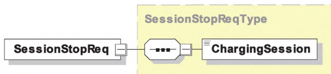
Рисунок 43 — Диаграмма — SessionStopReq
