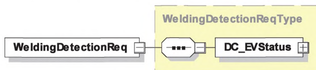
Рисунок 55 — Диаграмма — WeldingDetectionReq
