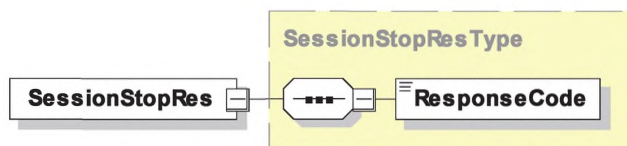
Рисунок 44 — Диаграмма — SessionStopRes
