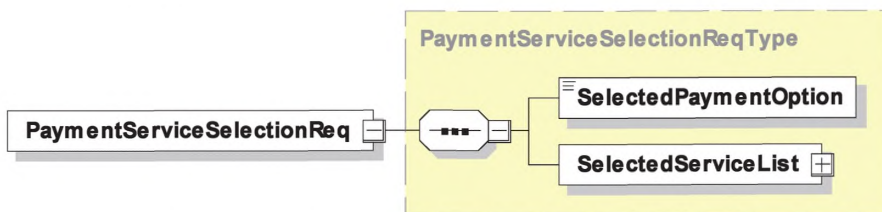
Рисунок 29 — Диаграмма — PaymentServiceSelectionReq
