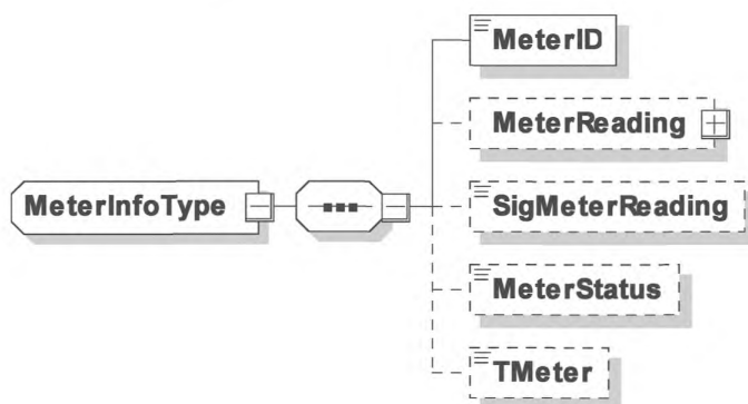
Рисунок 62 — Диаграмма — MeterInfoType
