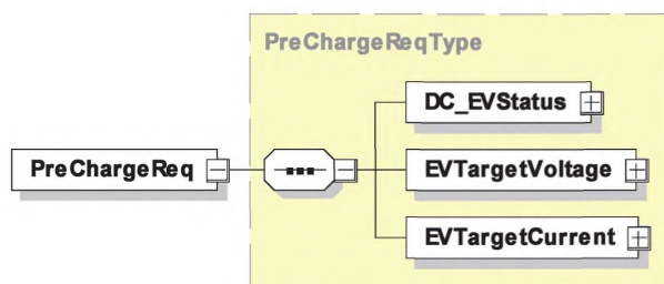
Рисунок 51 — Диаграмма — PreChargeReq
