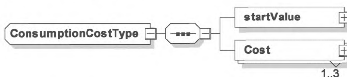
Рисунок 75 — Диаграмма — ConsumptionCostType
