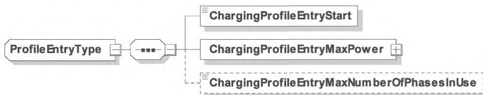
Рисунок 67 — Диаграмма — ProfileEntryType
