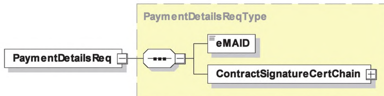
Рисунок 31 — Диаграмма — PaymentDetailsReq
