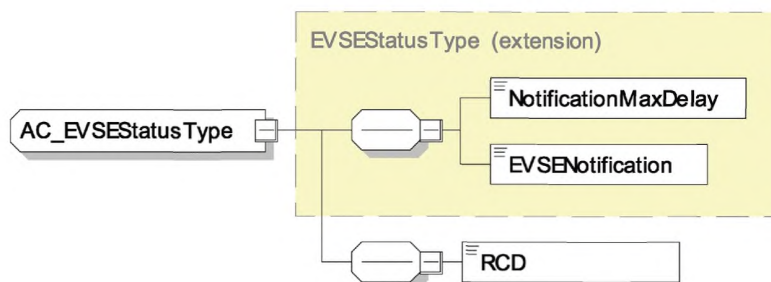
Рисунок 87 — Диаграмма — AC_EVSEStatusType
