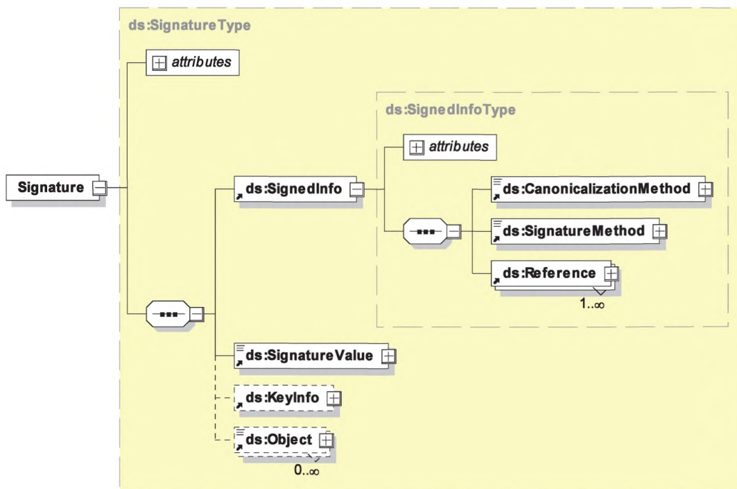
Рисунок 12 — Диаграмма — XML-подпись
