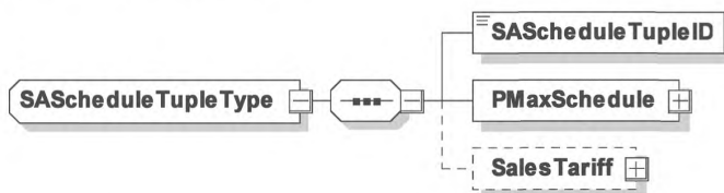
Рисунок 69 — Диаграмма — SAScheduleTupleType
