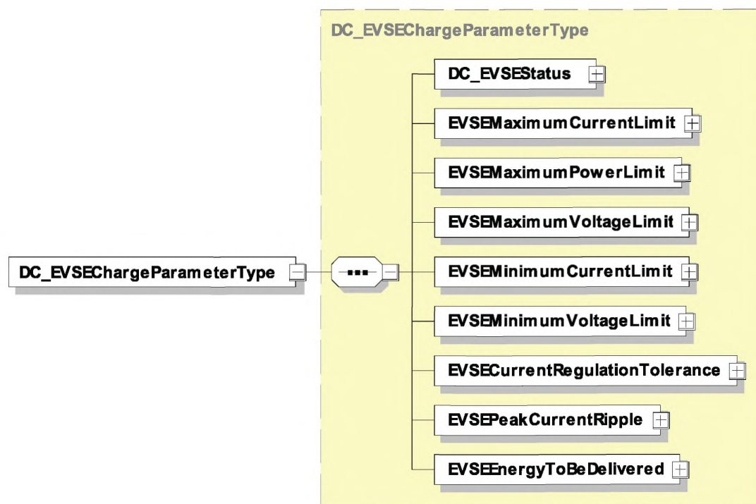
Рисунок 93 — Диаграмма — DC_EVSEChargeParameterType
