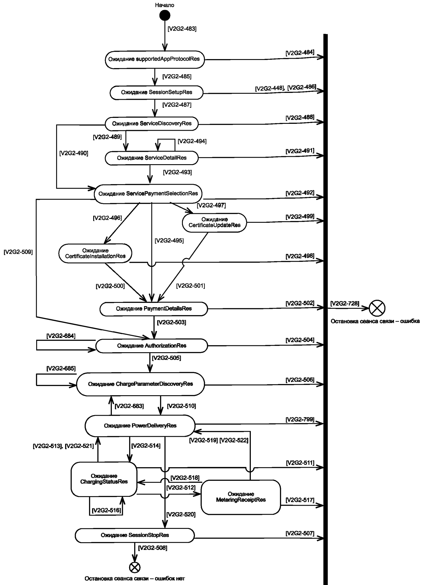
Рисунок 101 — Состояния связи EVCC для сообщений V2G при зарядке переменным током
