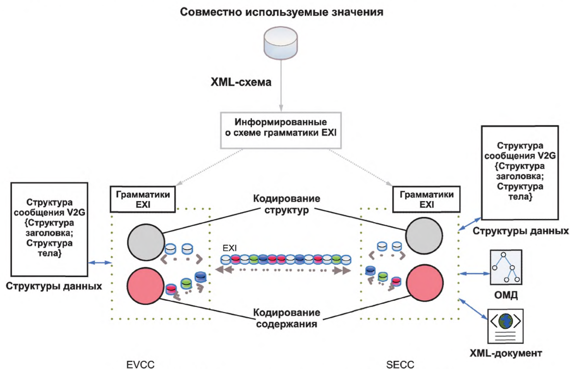
Рисунок 11 — Применение базовой концепции EXI к связи V2G
