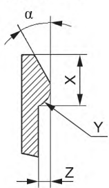
Деталь а
