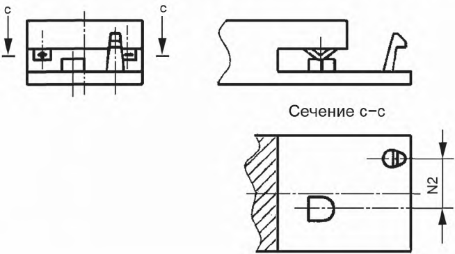
Единичный модульный соединитель с фиксатором -2. Остальные размеры указаны выше.
