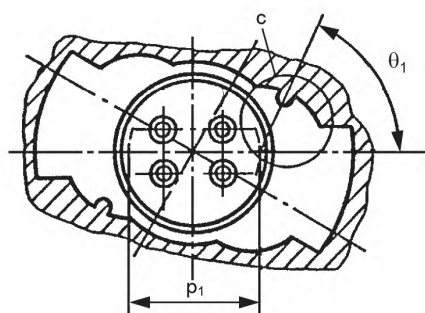
Сечение IV-IV, см. примечание (8)
