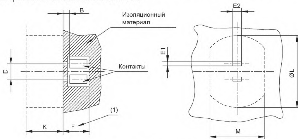
Рисунок 1 — Соединитель
