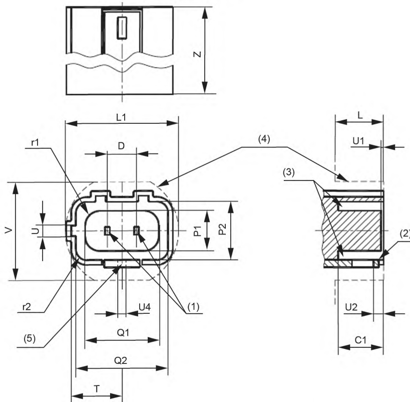
Соединитель PG20
