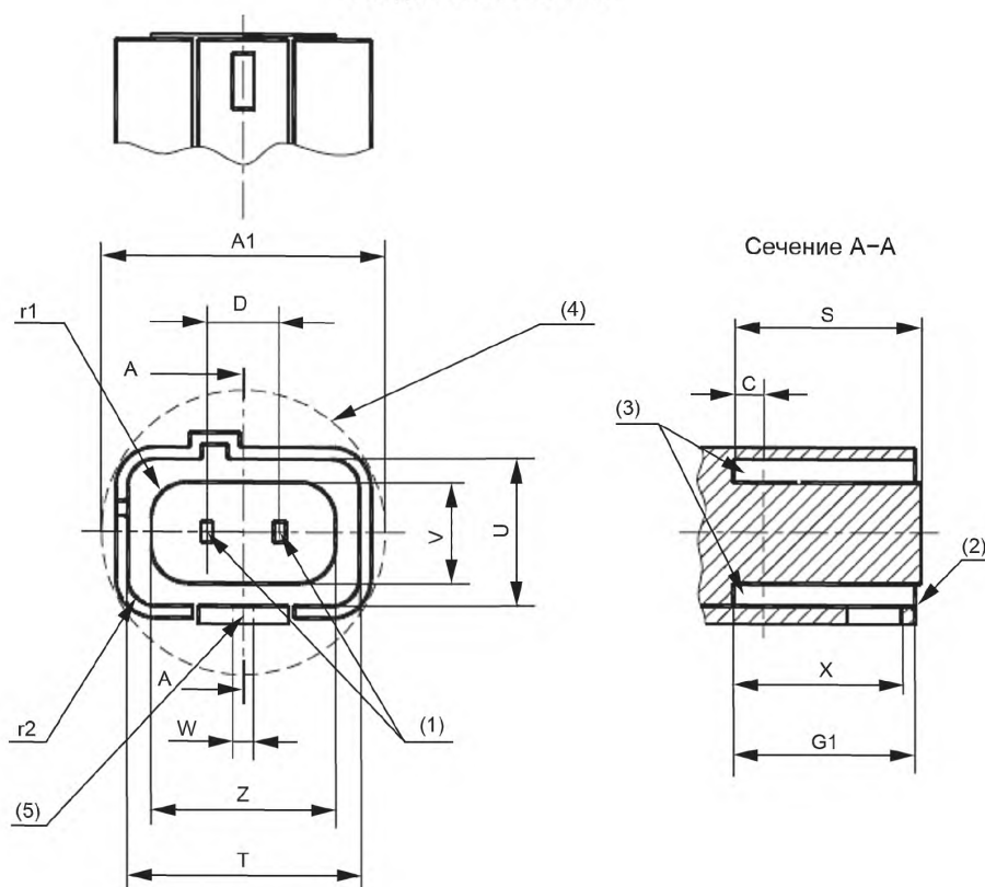
Соединитель PG18.5d
