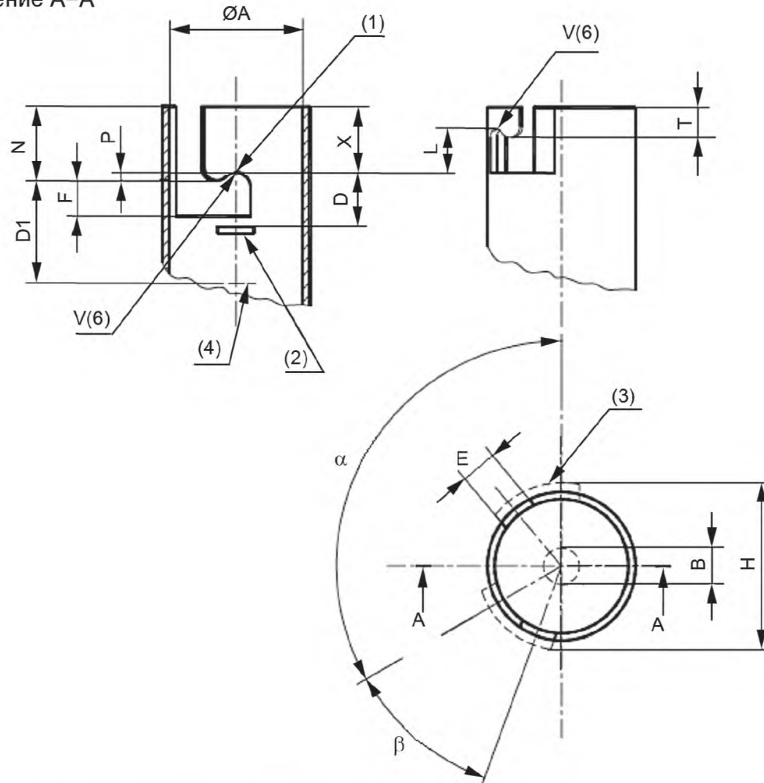
Сечение А-А
