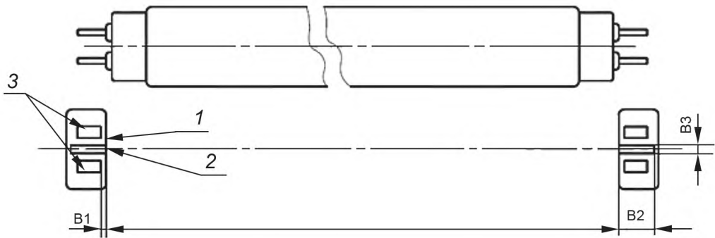
1 — патрон; 2 — входные пазы для штырьков; 3 — контакты
