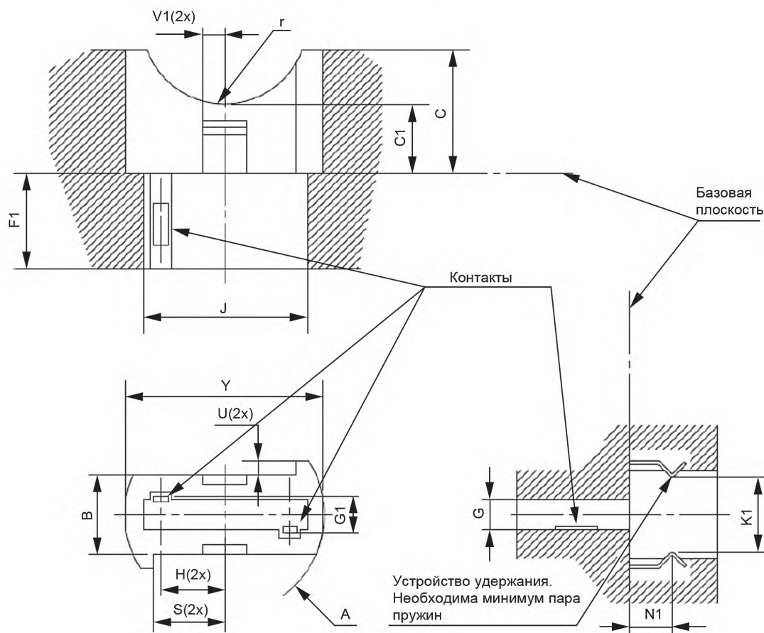
Форма базового паза
