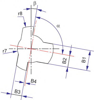
Монтажное отверстие
