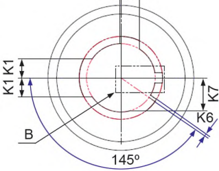
Рисунок 2, лист 1 — Размеры фиксаторов
