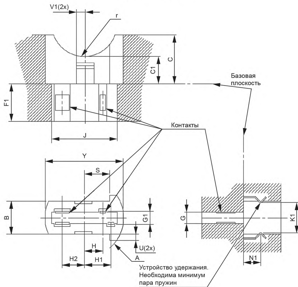
Форма базового паза
