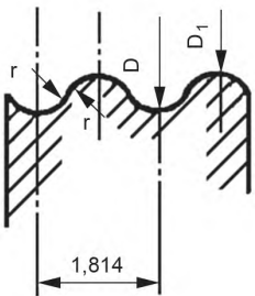
Деталь резьбы Правая резьба
