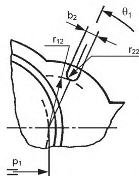
Сечение II-II
