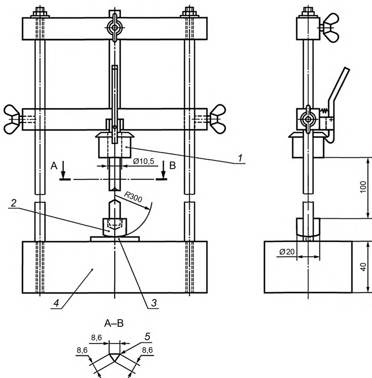
Разрез А-В
