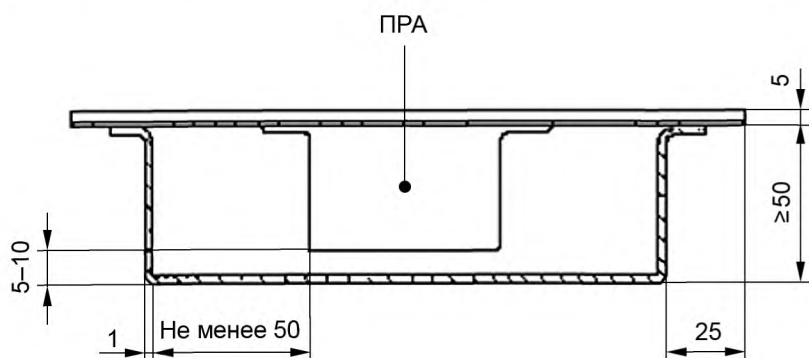
Рисунок J.1 — Испытательный кожух для тепловых испытаний ПРА
