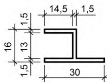
Рисунок В.1 — Профиль ПС 885-265
