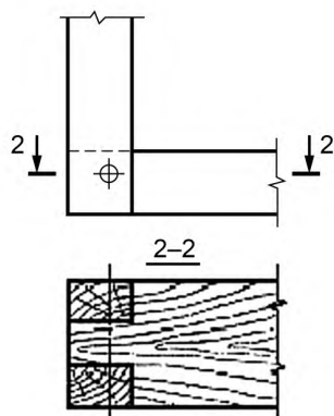
Рисунок Б.2 — Каркас с элементами сплошного сечения
