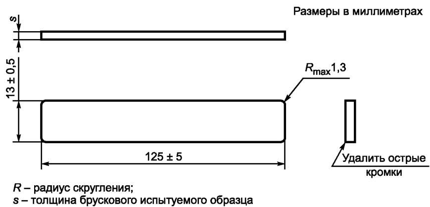
а – брусковый испытуемый образец
