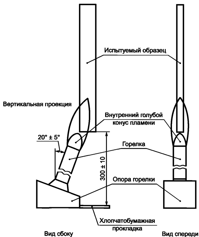
Рисунок 1 — Испытание вертикального горения для брускового испытуемого образца
