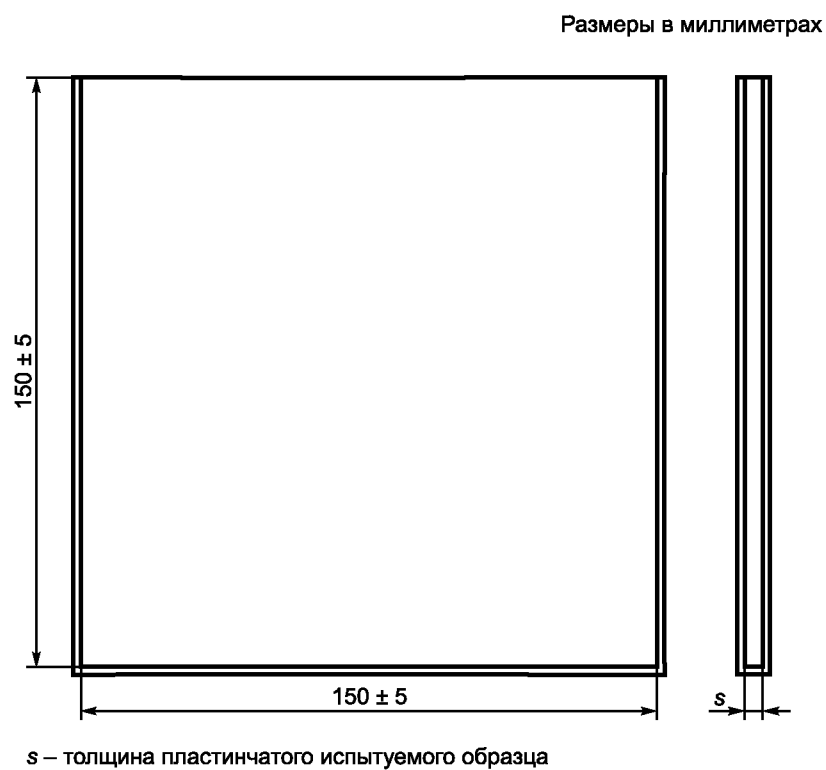
б – пластинчатый испытуемый образец
