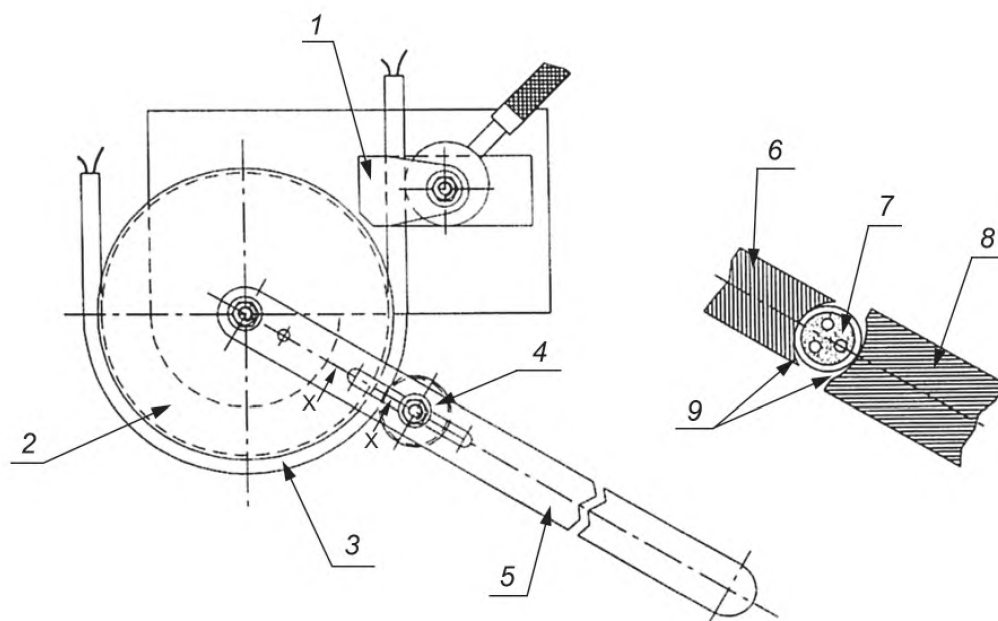
1 — зажим; 2 — оправка; 3 — кабель; 4 — ролик; 5 — рычаг для изгибания; 6 — оправка; 7 — кабель; 8 — ролик; 9 — радиус канавок; x — x — фрагмент в увеличенном масштабе
