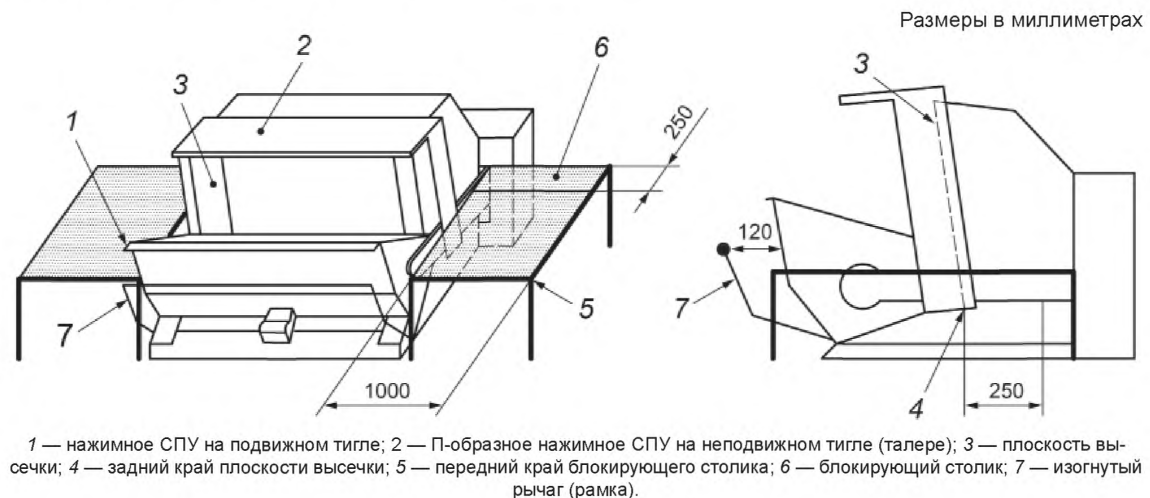
Рисунок 1 — Блокирующие столики
