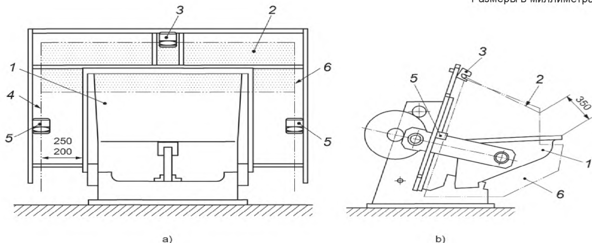
Рисунок 2 — Тигельная печатная машина, оборудованная лазерным сканером
