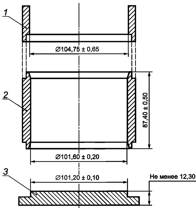
1 — удлинительное кольцо; 2 — цилиндрическая часть формы; 3 — основание формы
