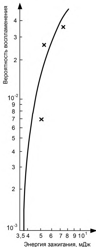
Рисунок 39.2 — Зависимость вероятности воспламенения пылевоздушной смеси сополимер СМЕД (ГОСТ 12271) от значения энергии зажигания
