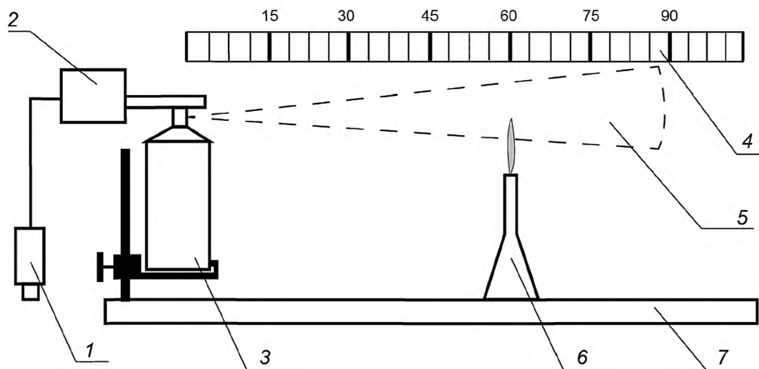
1 — кнопка управления устройством нажатия; 2 — устройство для нажатия на клапан аэрозольной упаковки; 3 — испытательная аэрозольная упаковка; 4 — измерительная линейка; 5 — струя аэрозоля; 6 — газовая горелка; 7 — основание для крепления
