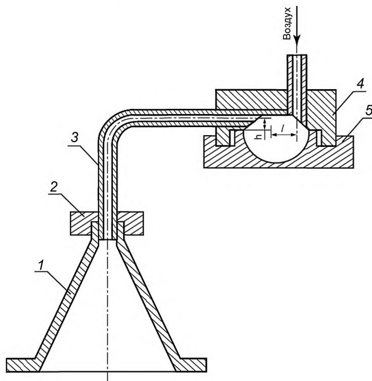
1 — конус; 2 — гайка накидная; 3 — патрубок; 4 — форкамера; 5 — донышко; h = l = 15,0 \pm 0,5
