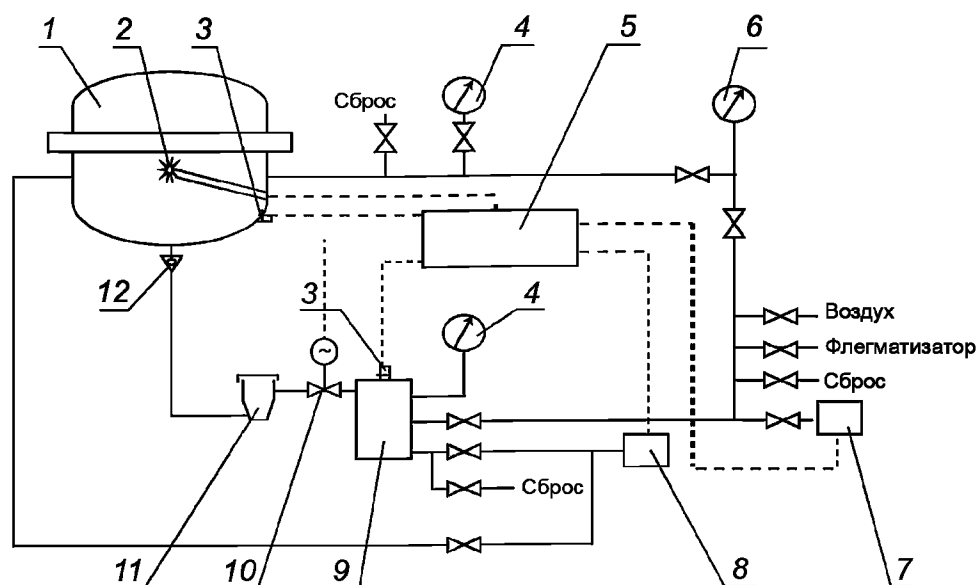
1 — реакционная камера; 2 — источник зажигания; 3 — датчики давления; 4 — манометры; 5 — блок управления и регистрации; 6 — вакуумметр; 7 — вакуумный насос; 8 — газоанализатор; 9 — ресивер; 10 — клапан мембранный с электромагнитным приводом; 11 — форкамера; 12 — обратный клапан
