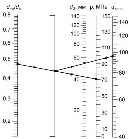
Рисунок 4 — Номограмма для определения диаметра заряда ФТ типа ТШТ для обрыва стальных бурильных труб в закрепленном трубами интервале
