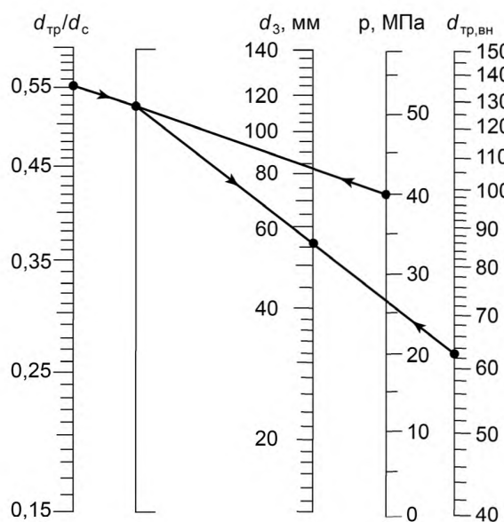
Рисунок 3 — Номограмма для определения диаметра заряда ФТ типа ТШТ для обрыва стальных бурильных труб в не закрепленном трубами интервале
