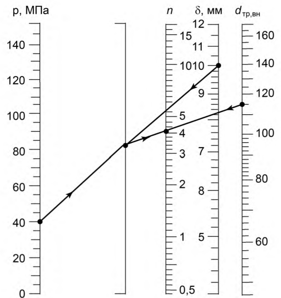
Рисунок 2 — Номограмма для определения числа ниток ДШ ФТ типа ТШ при ликвидации прихватов бурильных труб из алюминиевого сплава Д16Т
