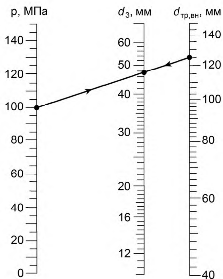
Рисунок 5 — Номограмма для определения диаметра заряда ФТ типа ТШТ для обрыва бурильных труб из алюминиевого сплава
