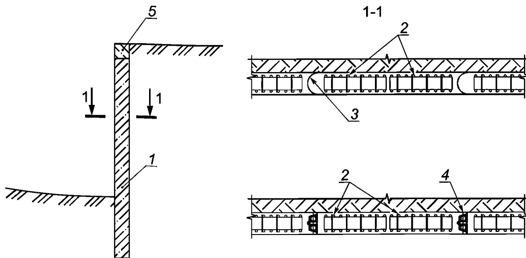
1 — «стена в грунте»; 2 — армирующий каркас; 3 — ограничитель захваток полукруглого типа; 4 — ограничитель захваток с гидрошпонкой; 5 — обвязочная балка
