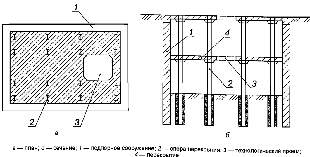
Рисунок 7.3 — Схема устройства котлована способом «сверху вниз»
