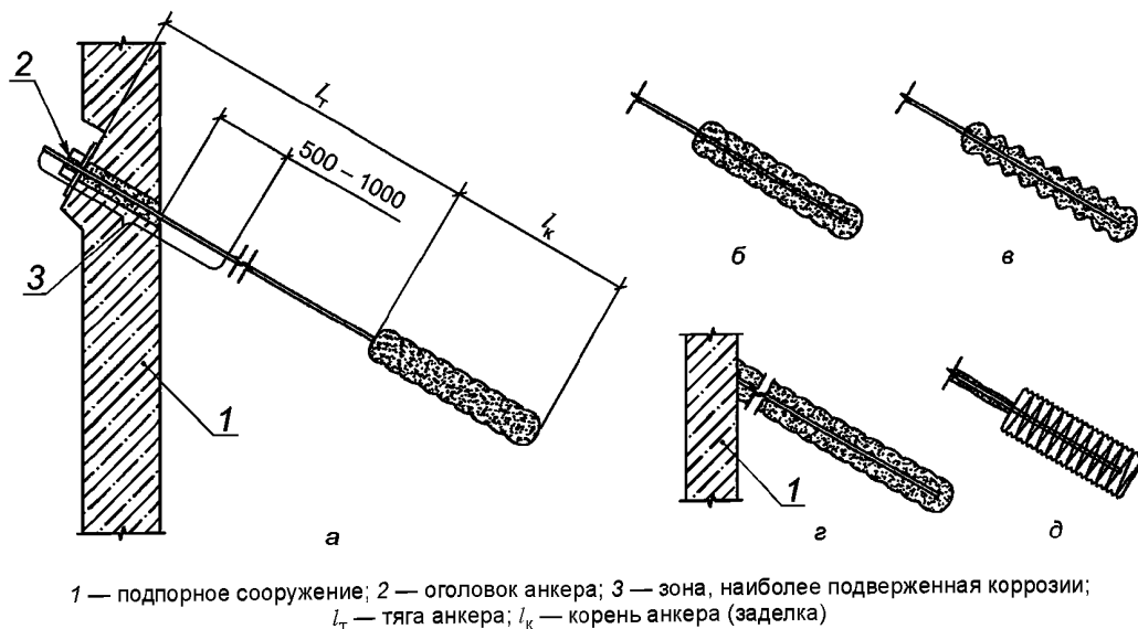
Рисунок 7.10 — Схема конструктивных элементов анкера (а) и форма его корней в зависимости от способа изготовления: б — инъекционные; в — анкеры РИТ; г — анкеры с теряемой буровой штангой; д — анкеры с теряемой буровой штангой с корнем, выполняемым по струйной технологии
