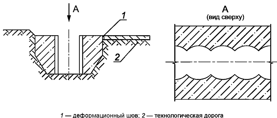
Рисунок 8.7 — Пример конструкции форшахты подпорного сооружения из буресекущихся свай
