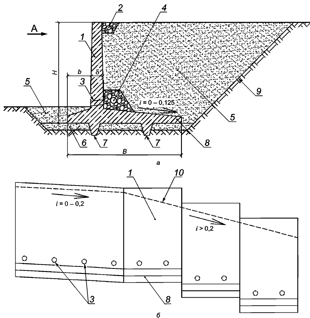
а — поперечное сечение; б — вид спереди (вид А); 1 — лицевая стенка; 2 — водоотводной кювет; 3 — дренажные трубки (шаг — 3—6 м); 4 — пристенный дренаж; 5 — обратная засыпка; 6 — подготовка основания «постель»; 7 — «зуб»; 8 — фундаментная плита; 9 — контур траншеи; 10 — контур поверхности земли; i — уклон
