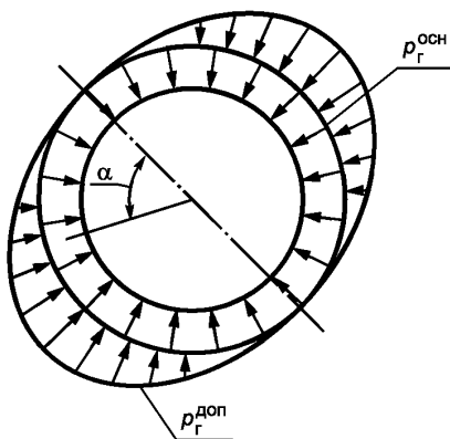
Рисунок 6.2 — Схема неравномерного распределения давления грунта на подпорное сооружение круглой формы в плане
