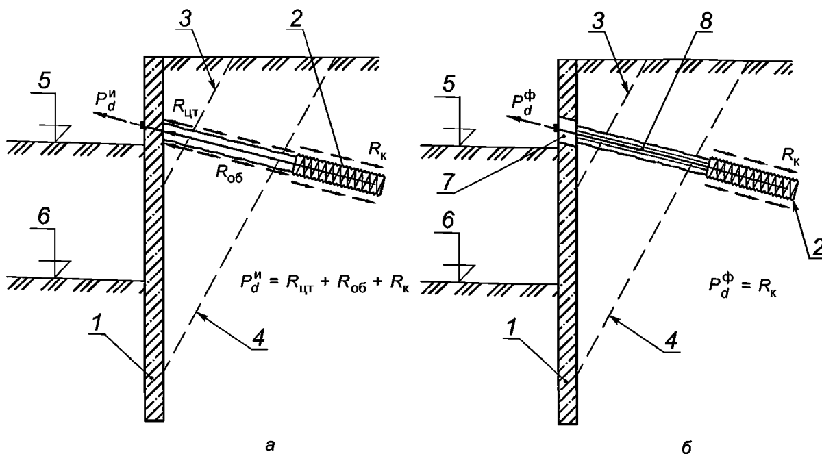
Рисунок 8.11 — Винтовая штанга
