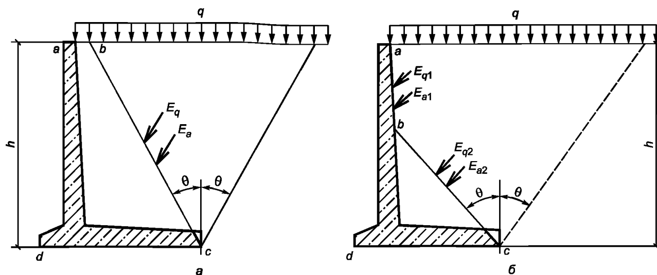
а — при симметричной призме обрушения; б — при короткой консоли и несимметричной призме обрушения; Eq_1, Eq_2 — горизонтальная составляющая давления от поверхностной нагрузки выше и ниже точки b соответственно; Ea_1, Ea_2 — горизонтальная составляющая активного давления выше и ниже точки b соответственно
