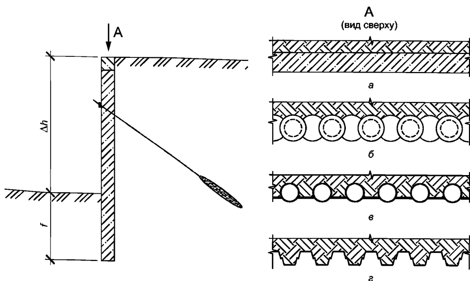
а — траншейная железобетонная «стена в грунте»; б — ограждение из буровых свай; в — ограждение из металлических труб с заборкой; г — шпунтовое ограждение типа «Ларсен»; \Delta h — перепад высот; f — зона заделки
