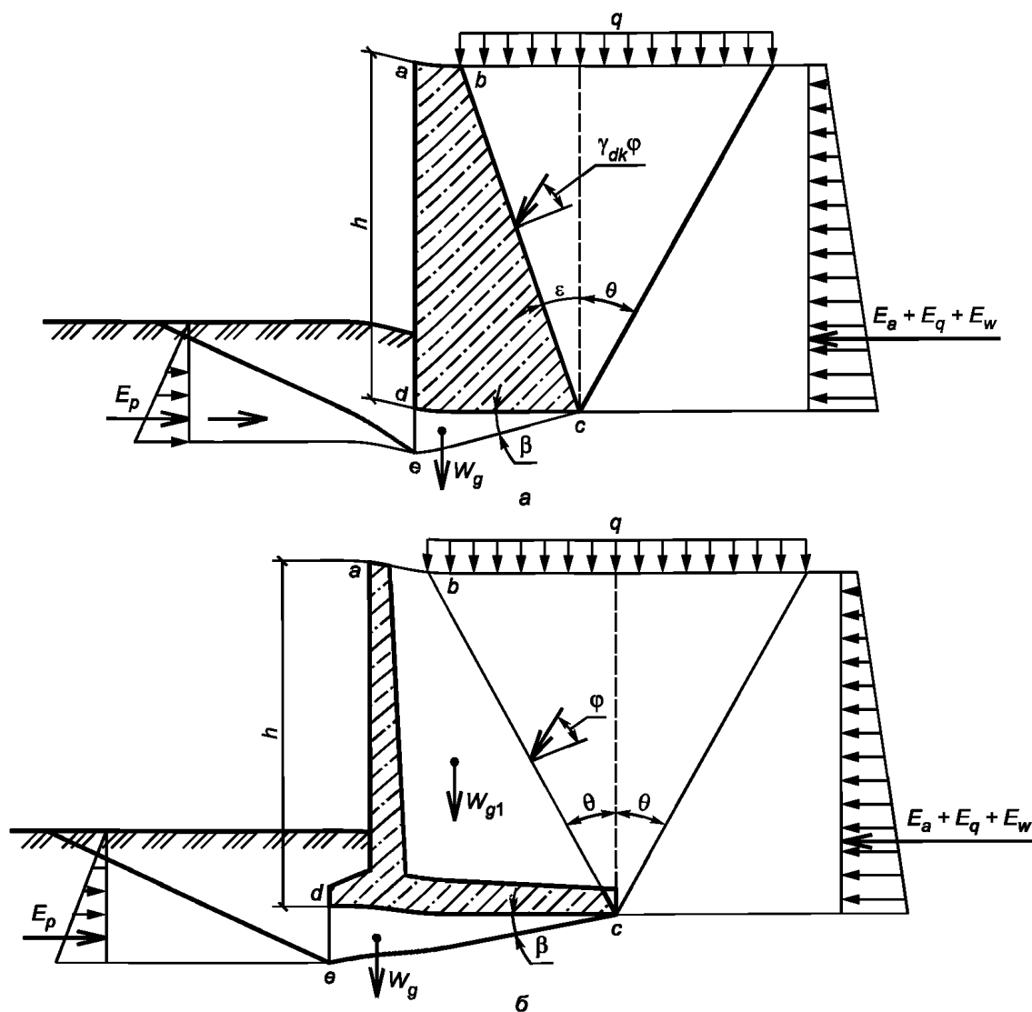
а — массивных стен; б — уголковых стен; W_{g1} — равнодействующая веса грунта в объеме abcd ; W_g — равнодействующая веса грунта в объеме cde ; \gamma_{dk\phi} — коэффициент условий работы на контакте; \beta — угол наклона поверхности скольжения к горизонту
