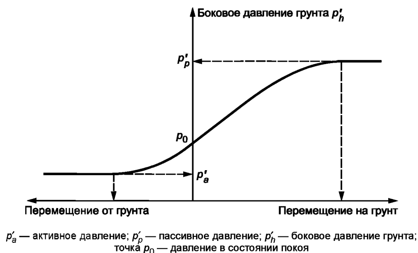
Рисунок 6.1 — Изменение давления грунта на подпорное сооружение в зависимости от его перемещения
