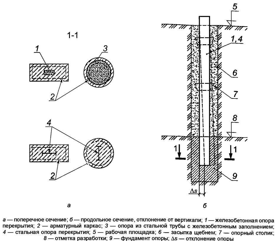
Рисунок 7.5 — Схема установки опоры для перекрытия
