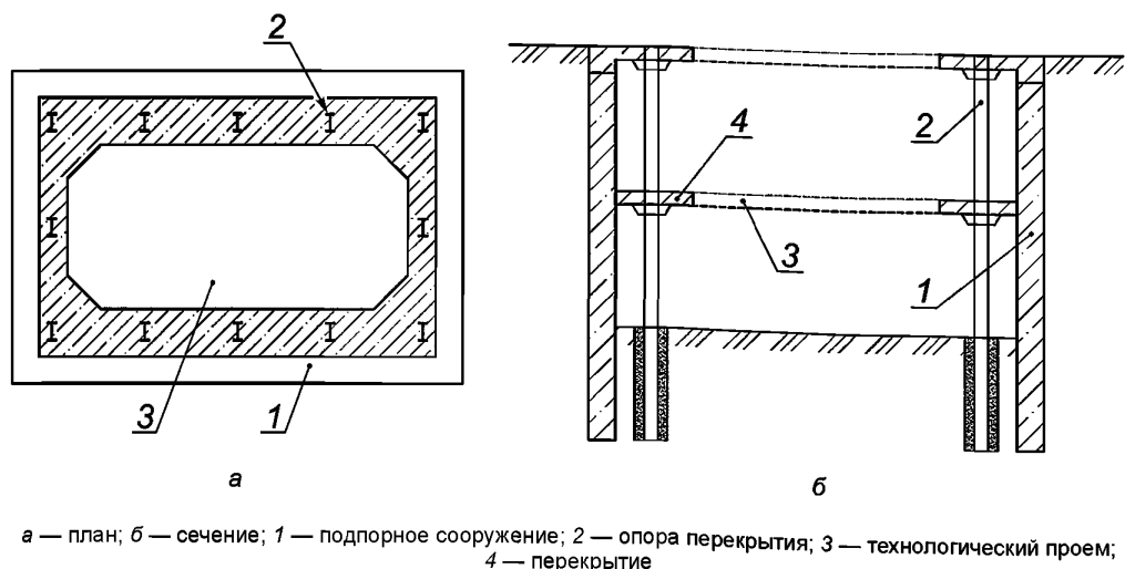
Рисунок 7.4 — Схема устройства котлована способом «сверху вниз» по периметру котлована
