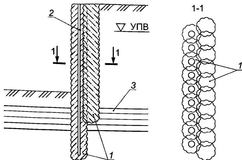
Рисунок Г.8 — Подпорное сооружение из грунтоцементных элементов в два ряда
