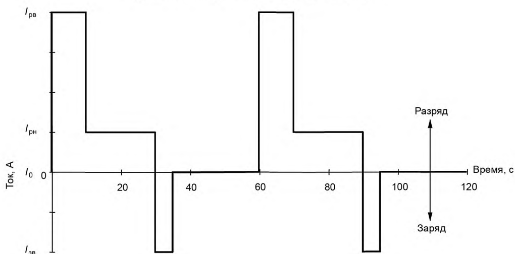
Динамический режим разряда с рекуперацией
