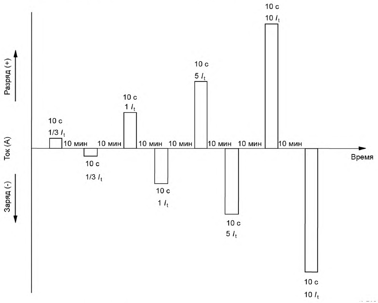
Рисунок А.3 — Порядок получения вольт-амперной характеристики (пример с испытываемыми аккумуляторами с нормированной емкостью менее 20 А·ч)
