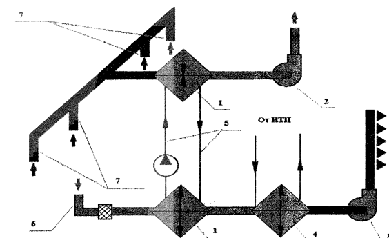
Рис. 7.1 Местная система вентиляции с теплоутилитатором
