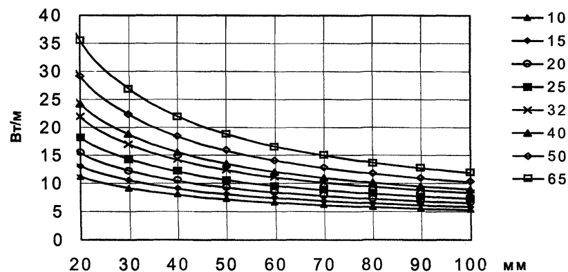
Рис. П. 8. Ориентировочные значения тепловых потерь для подающих трубопроводов систем отопления и горячего водоснабжения при коэффициенте теплопроводности тепловой изоляции 0,03 Вт/(м·°C)
