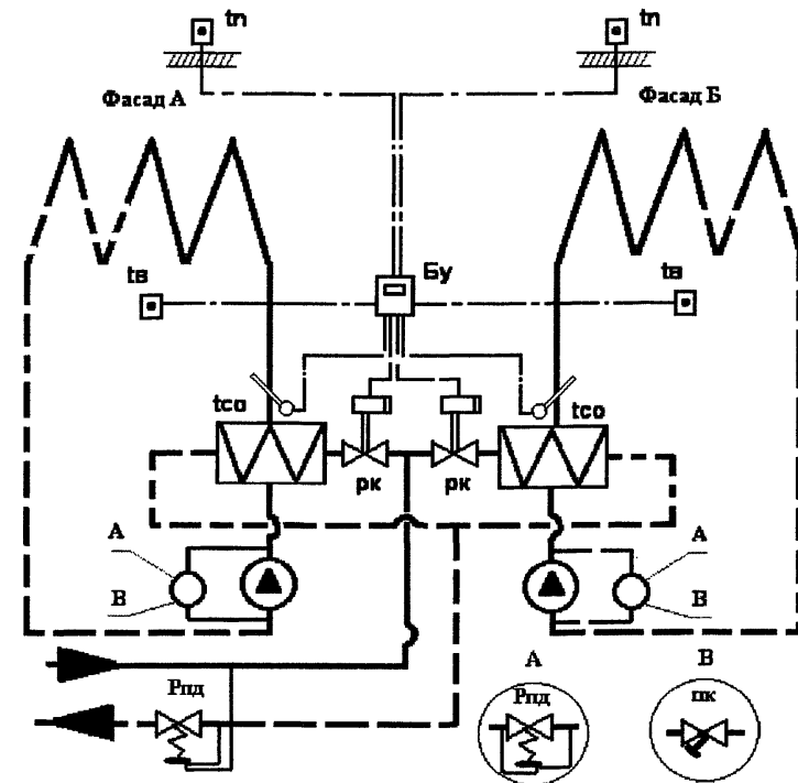
Рис. 8.18. Схема пофасадной автоматизации при независимом подключении СО
