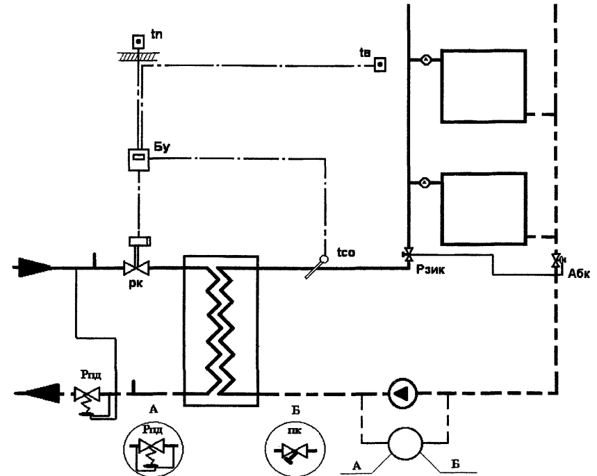
Рис. 8.9. Схема автоматизация теплового пункта с независимым присоединением СО
