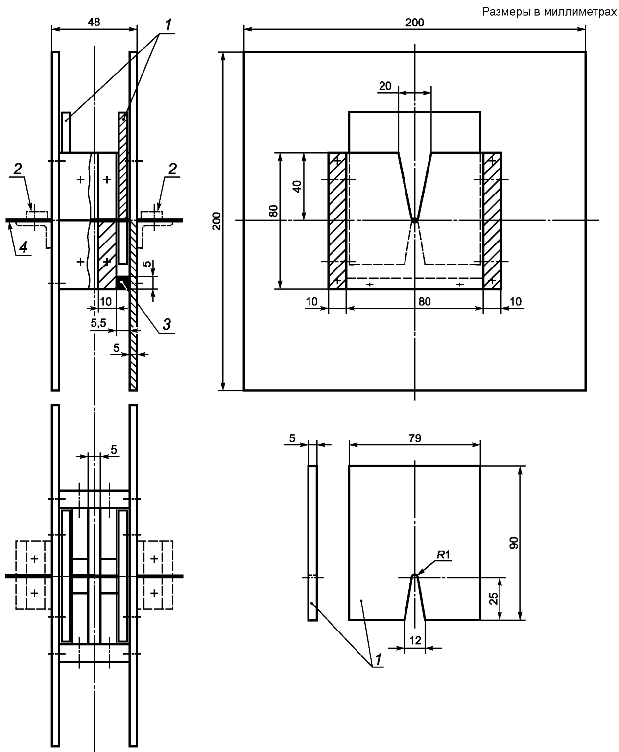
Рисунок 105 — Испытательная установка для проверки минимальных значений I_{ct} и I_p , выдерживаемых разъединителем
