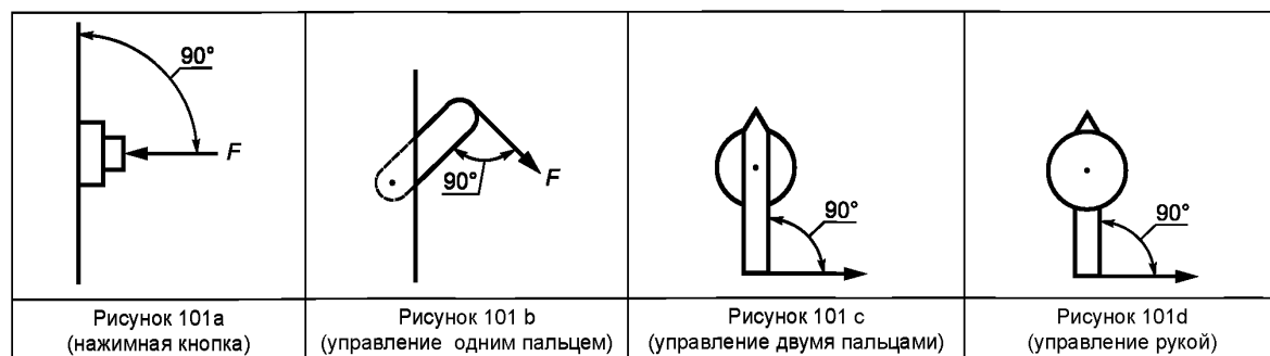
Рисунок 101 — Усилие F , применяемое к органу управления
