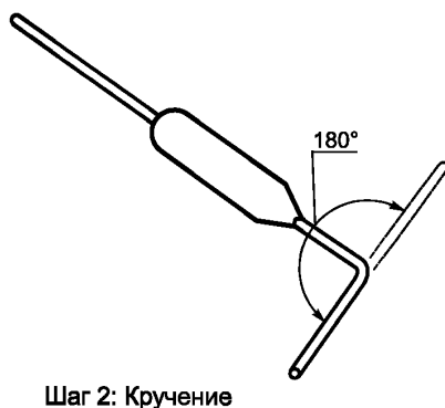
Рисунок 1 — Изгибающая/скручивающая сила
