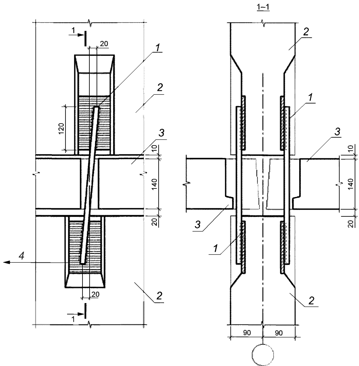
1 — вертикальная связь; 2 — внутренняя стеновая панель; 3 — плита перекрытия; 4 — направление расположения наружной стены
