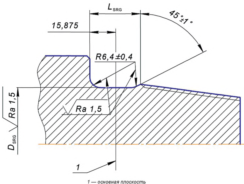
Рисунок 8 — Разгрузочная расточка на муфтовом конце
