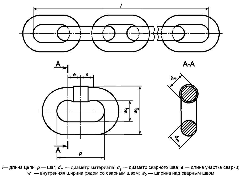
Рисунок 1 — Размеры звена и цепи
