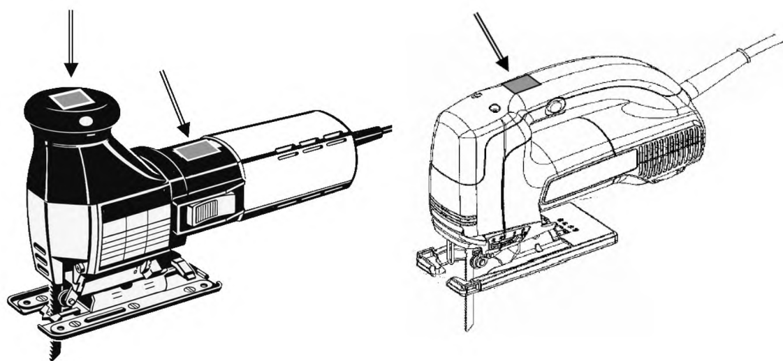
Рисунок I.104 — Расположение измерительных преобразователей для лобзиков
