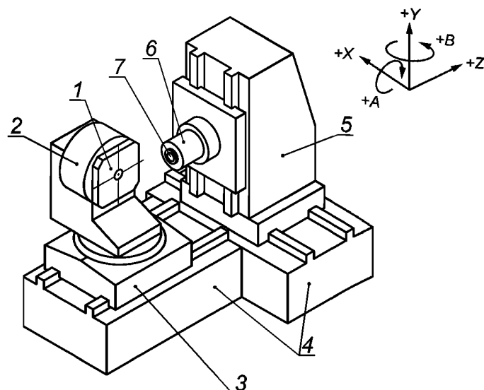
1 — поворотный стол (ось A' ); 2 — стол с вертикальной осью поворота (ось B' ); 3 — салазки стола (ось Z' ); 4 — станина; 5 — стойка (ось X' ); 6 — шпиндельная головка (ось Y' ); 7 — шпиндель [ось ( C1 )]
