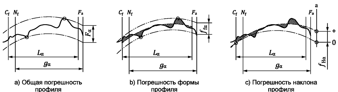
Рисунок 5 — Погрешности профиля с модифицированным углом зацепления
