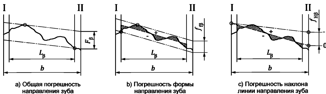
Рисунок 10 — Погрешности направления зуба с модификацией угла наклона зуба
