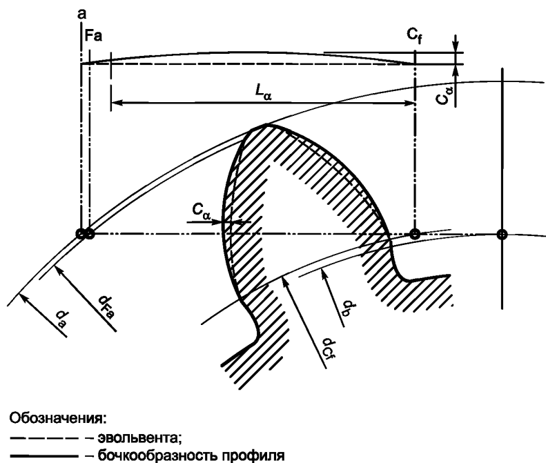
Рисунок В.1 — Бочкообразность профиля
