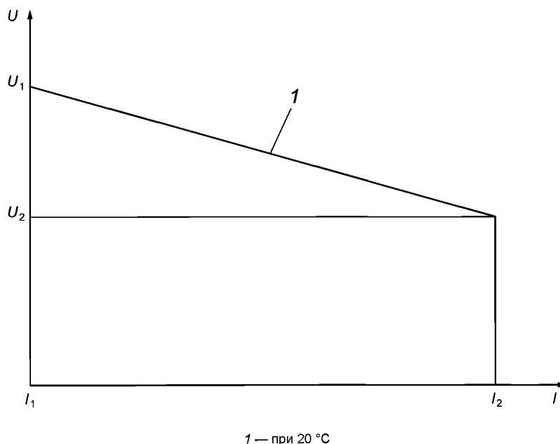
Рисунок 1 — Вольтамперная характеристика источника питания стартера
