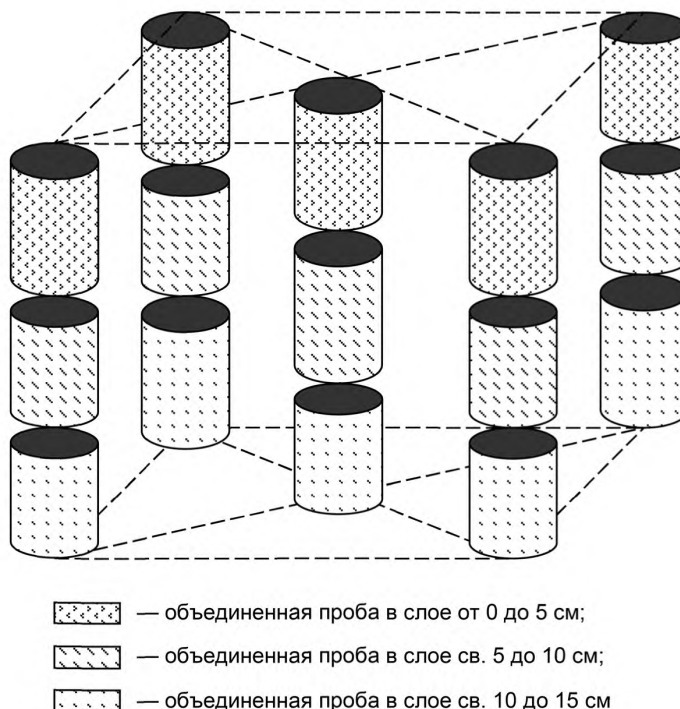
Рисунок 2 — Схема формирования объединенной пробы
