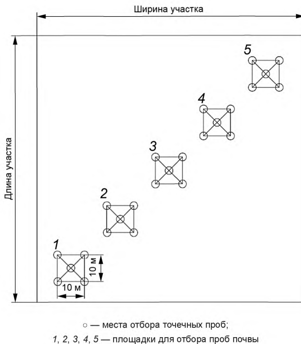
Рисунок 1 — Схема размещения площадок для отбора проб почвы
