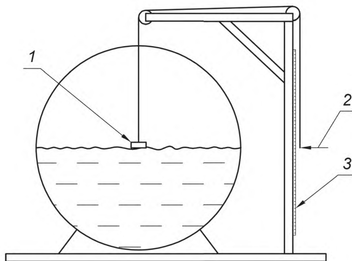
1 — поплавок; 2 — датчик; 3 — градуированная шкала
