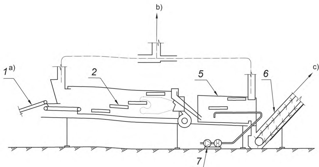
а) Сушильный барабан с отдельным смесительным барабаном
