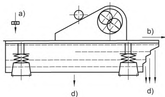
б) Вибрационный грохот с горизонтальной просеивающей поверхностью
