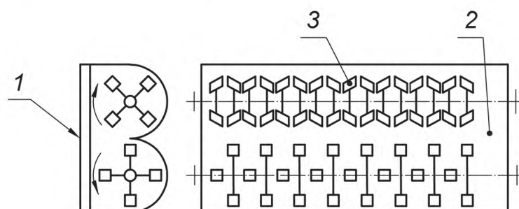
b) Двухвальный лопастной смеситель непрерывного действия
