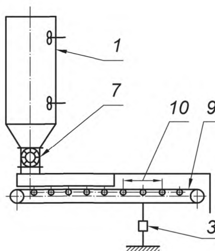
в) Непрерывного действия с весовой лентой
