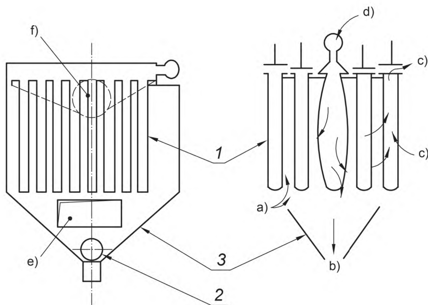
а) Со шнековым конвейером
