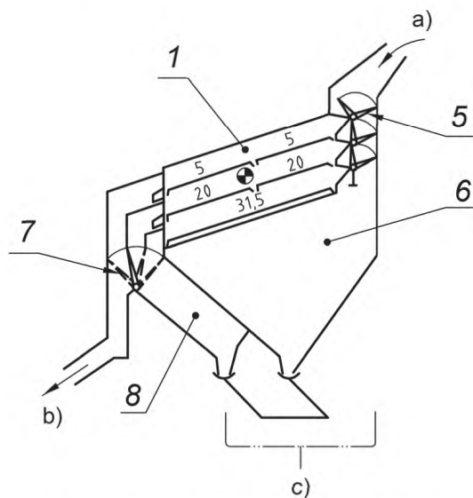
в) Стандартный классифицирующий грохот с тремя просеивающими поверхностями
