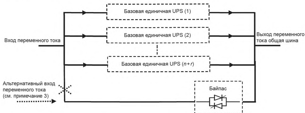
Рисунок А.3 — Параллельная UPS с общим байпас
