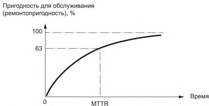
Рисунок К.2 — График зависимости пригодности для обслуживания, %, от времени
