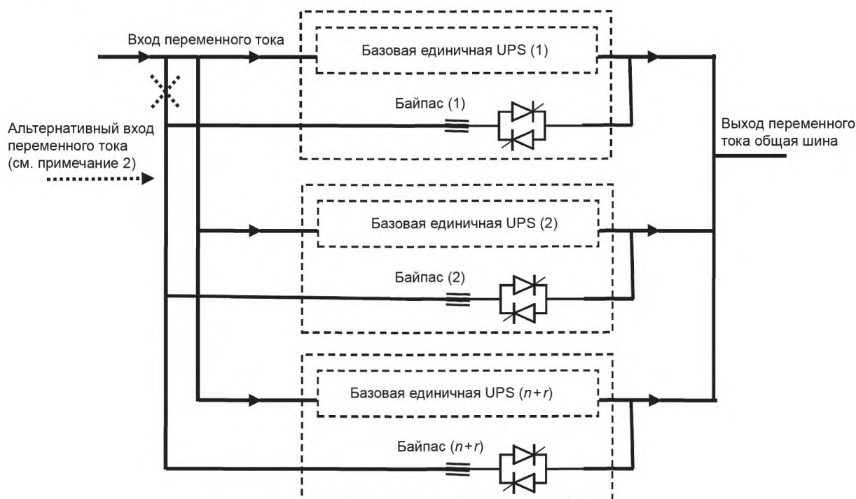
Рисунок А.4 — Параллельная UPS с распределенным байпас
