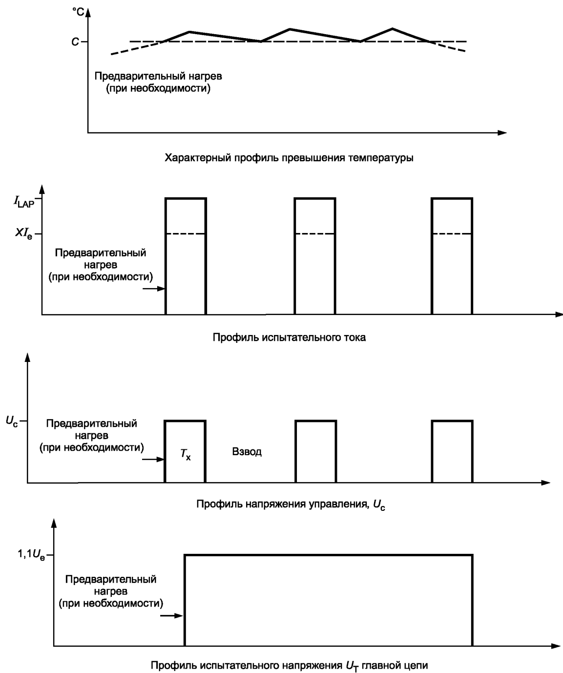
Рисунок F.2 — Профиль испытания на перегрузочную способность
