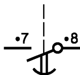
Замыкающий контакт с замедлением при замыкании
