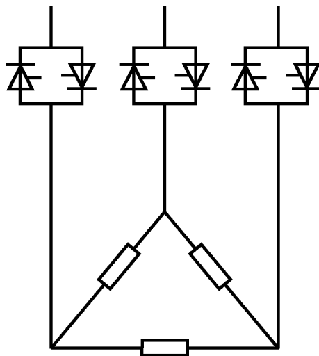
б — Нагрузка со схемой «треугольник», тиристоры между нагрузкой и питанием
