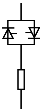
с — Однофазная нагрузка, тиристоры между нагрузкой и питанием
