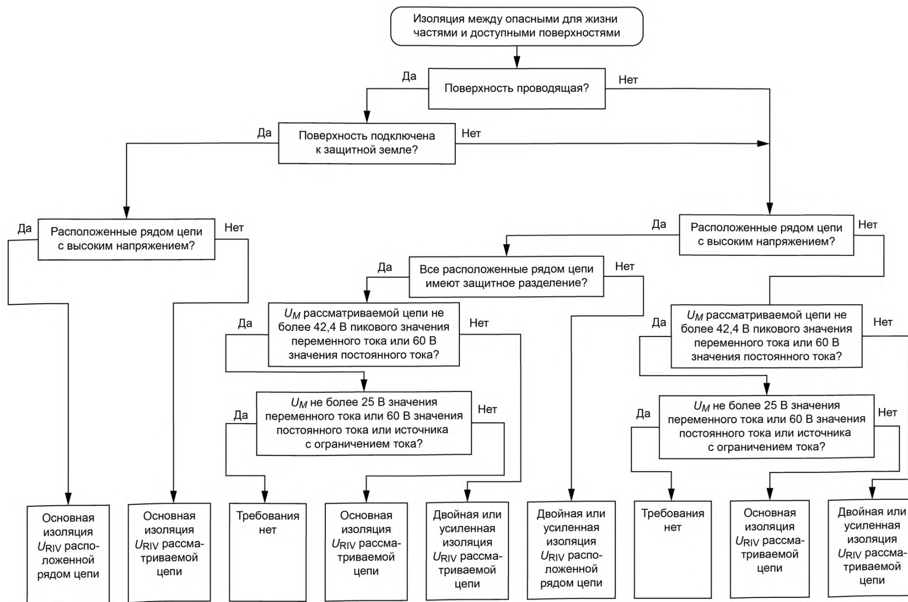
Рисунок 5 — Выбор изоляции между частями, находящимися под напряжением, и доступными поверхностями
