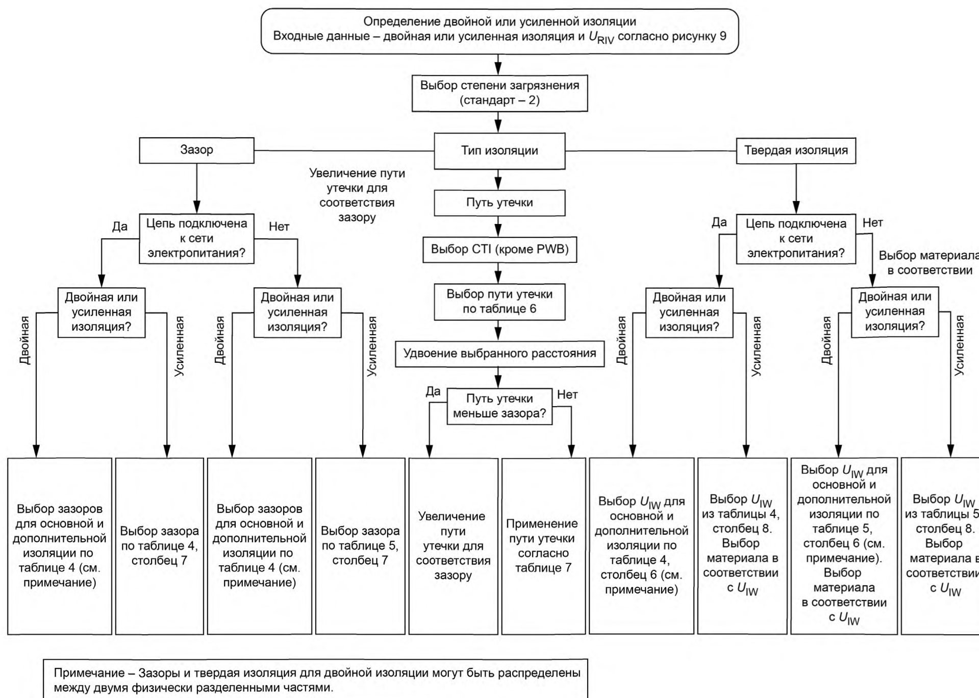
Рисунок 9 — Выбор двойной и усиленной изоляции
