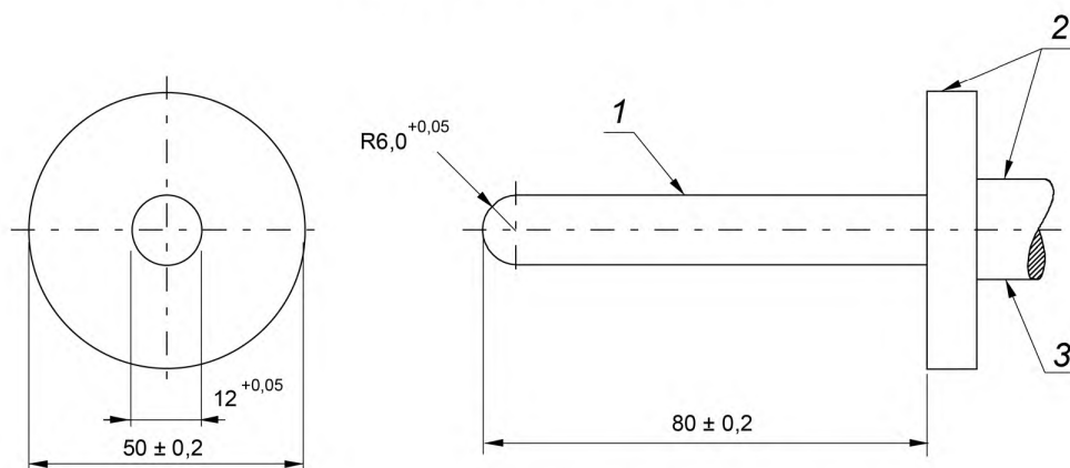
Рисунок 2 — Испытательный штырек
