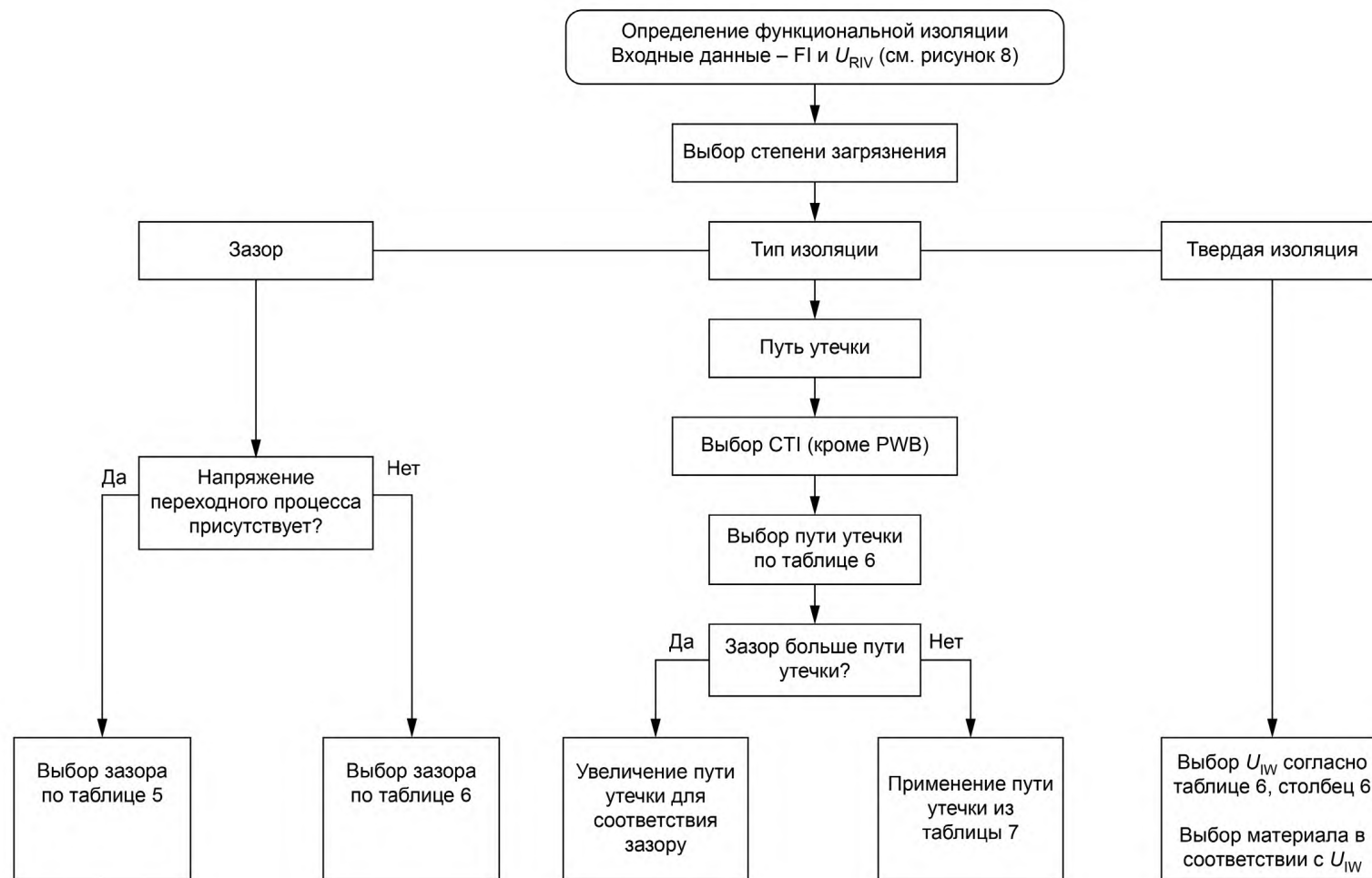
Рисунок 7 — Выбор функциональной изоляции
