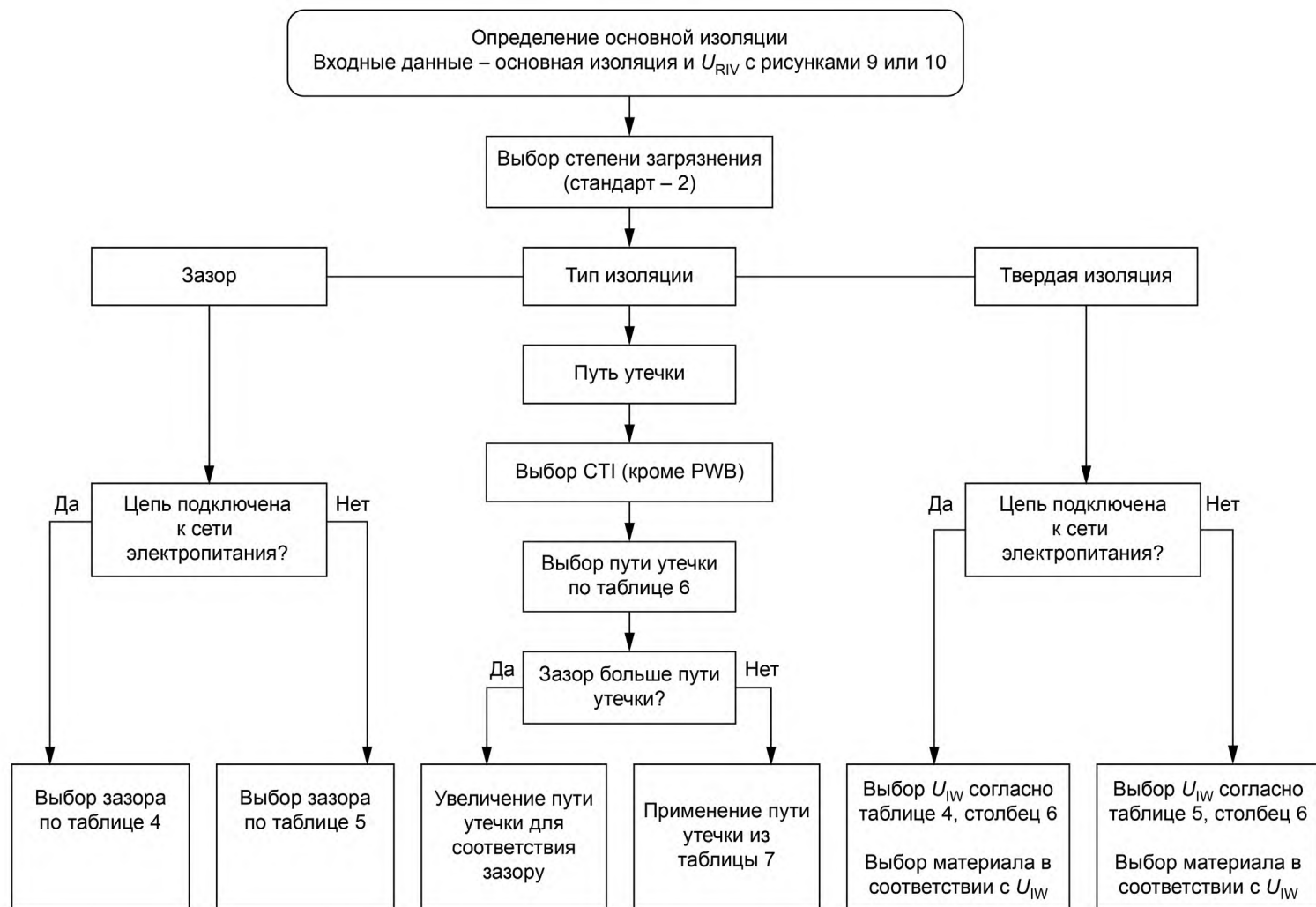
Рисунок 8 — Выбор основной изоляции
