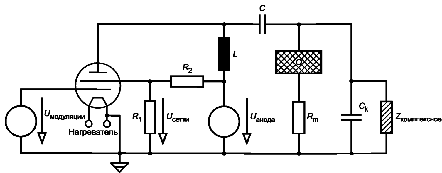
Рисунок D.2 — Высокочастотный генератор большой мощности [5] и [6]
