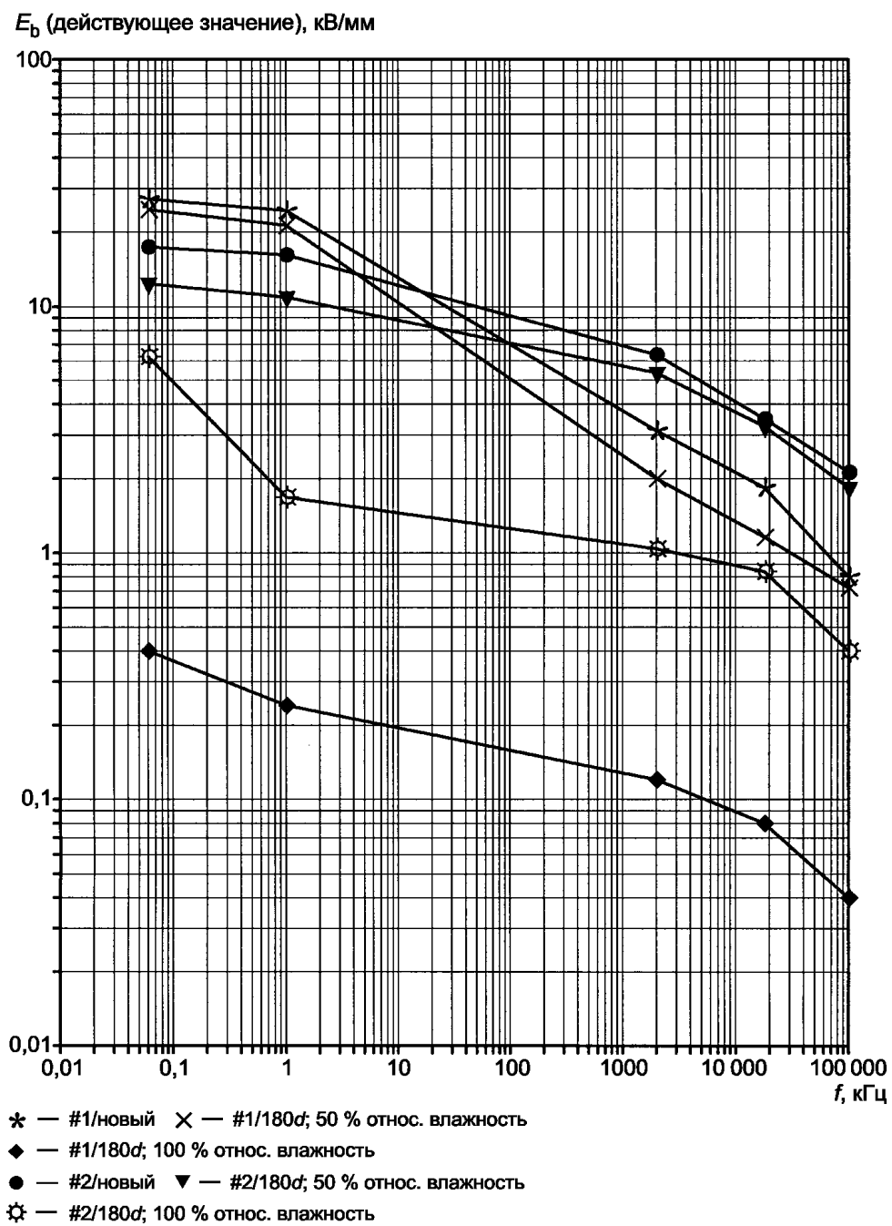
Рисунок С.4 — Высокочастотный пробой твердой изоляции, влияние влажности; условия при 50 °С: #1: наполненный слюдой фенол, d = 0,75 мм; #2: ламинат из кремниевое стекла, d = 0,75 мм [19]
