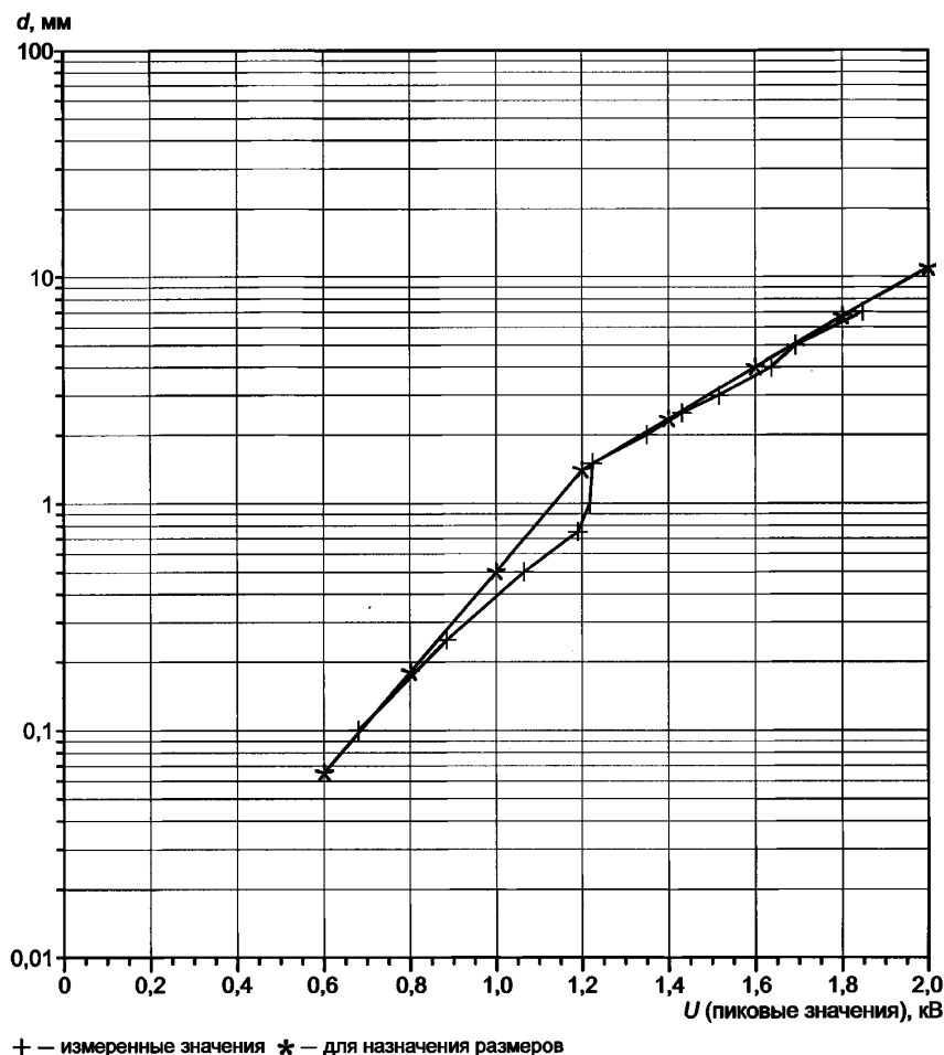
Рисунок 1 — Размеры воздушных промежутков в неоднородном поле в воздушной среде при атмосферном давлении (радиусы точек электродов в плане — 5 мкм) для исключения случаев ЧП или пробоев (воздушные зазоры менее 1 мм)
