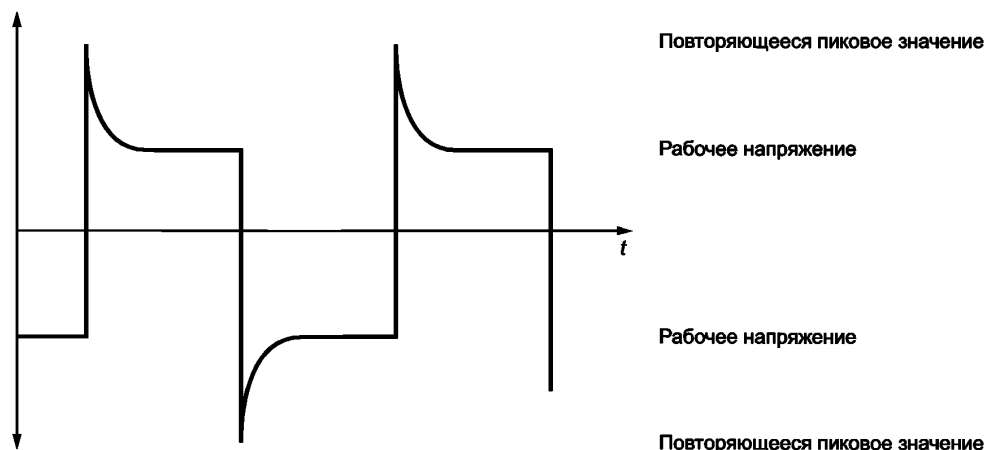
Рисунок 4 — Периодическое импульсное напряжения (см. IEC 60664-1)
