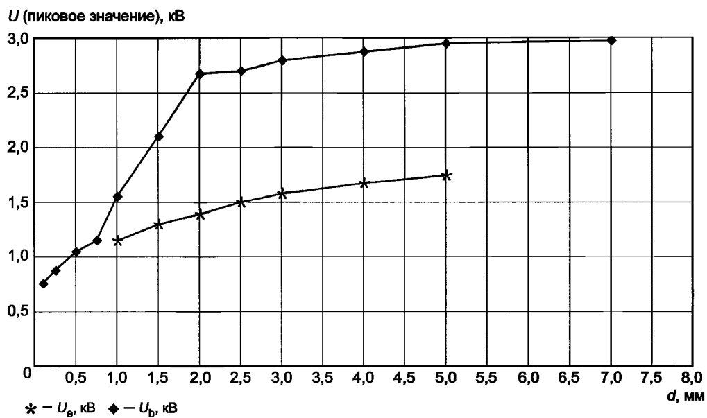
Рисунок А.5 — Напряжения затухания ЧП и напряжения пробоя в воздухе при атмосферном давлении для частоты 460 кГц, точечные электроды с ВВ-иглами [6]
