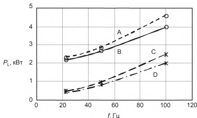
A — полная нагрузка, ШИМ-питание; B — полная нагрузка, синусоидальное питание; C — без нагрузки, ШИМ-питание; D — без нагрузки, синусоидальное питание
