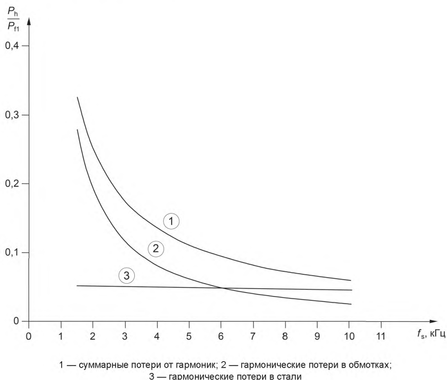
Рисунок 4 — Пример зависимости потерь в электрической машине, вызванных гармониками P_h относительно потерь P_{f1} , на рабочей частоте f_1 и частоте коммутации f_s в случае питания от двухуровневого инвертора напряжения
