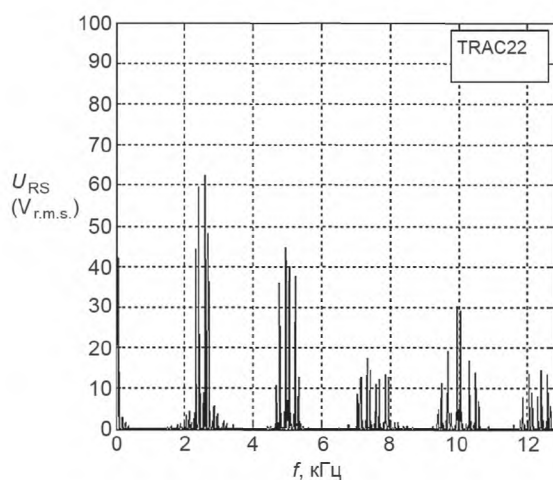
а — ШИМ на постоянной частоте
