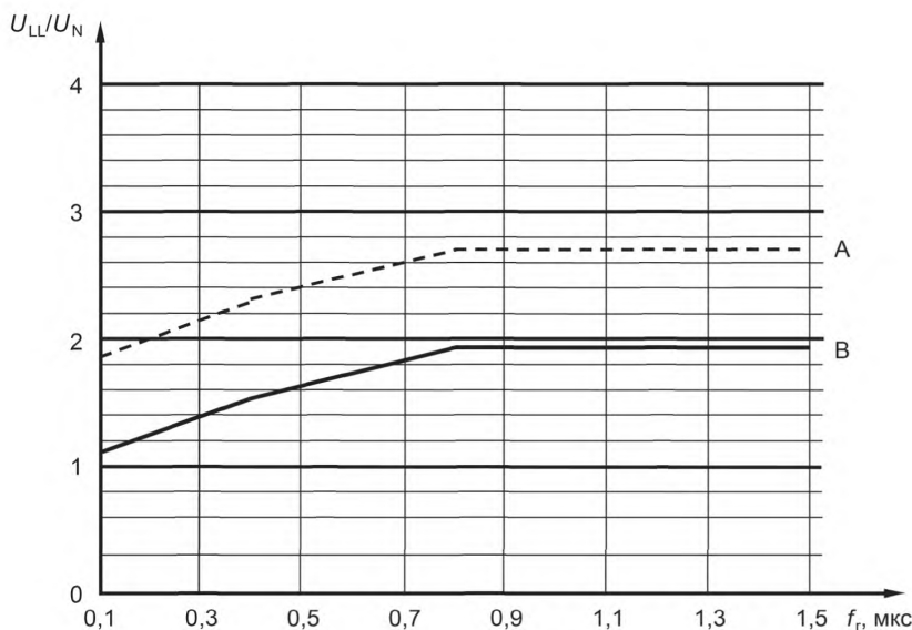
A — стандартные машины; B — машины со старой системой изоляции
