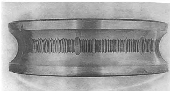
Рисунок 18 — Появление бороздок из-за чрезмерного тока в подшипниках
