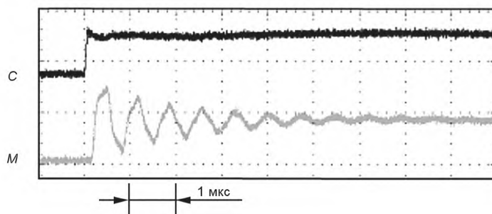
С — фазное напряжение преобразователя; М — фазное напряжение двигателя
