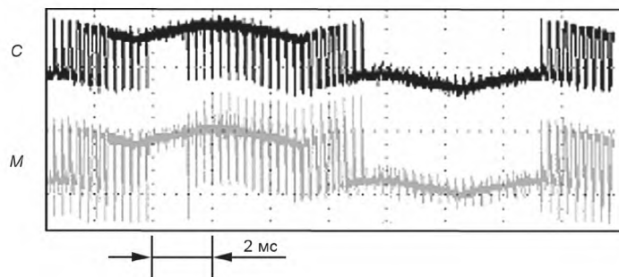
С — фазное напряжение преобразователя; М — фазное напряжение двигателя
