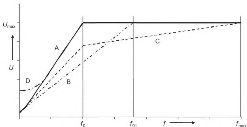
Рисунок 3 — Характеристики «выходное напряжение преобразователя — частота»
