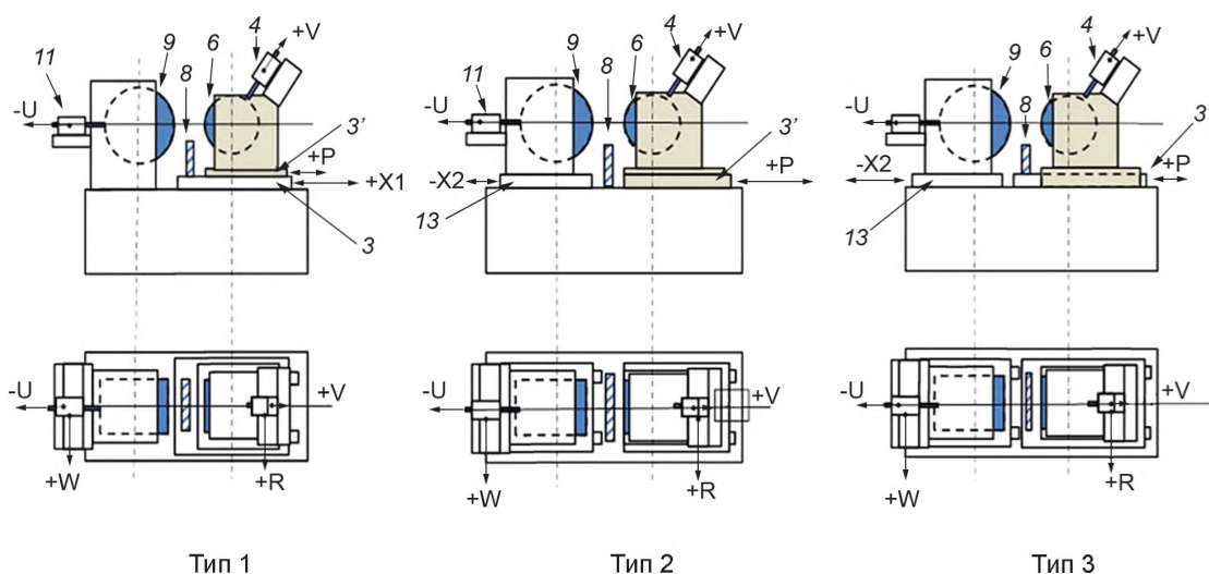
Рисунок 2 — Примеры конфигураций бесцентрового шлифовального станка
