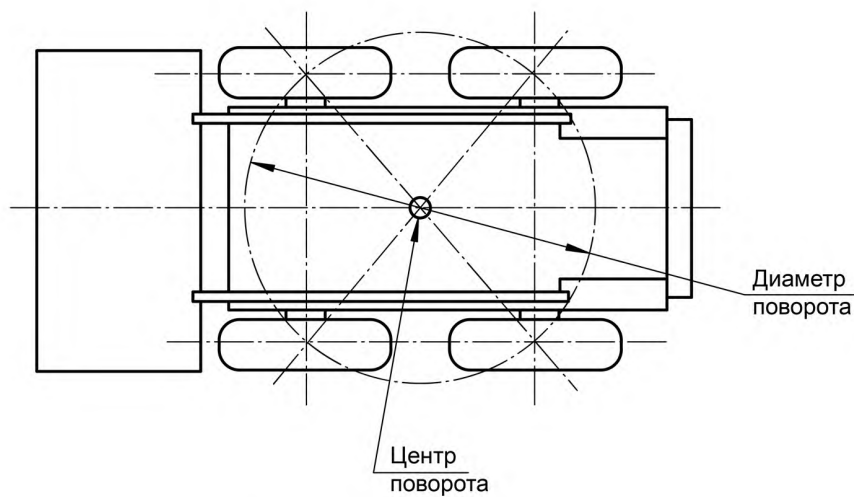
а) машина с бортовым поворотом
