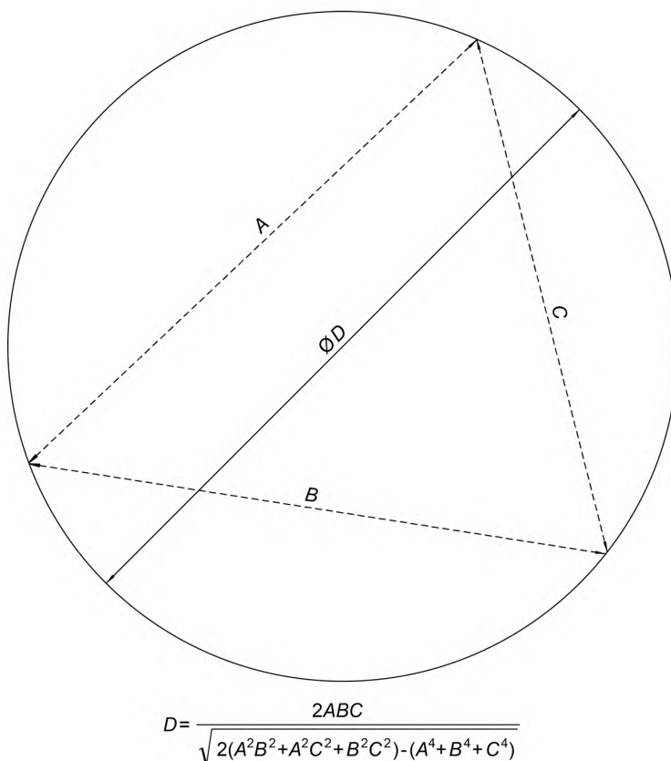
Рисунок 3 — Расчет диаметров по измеренным отрезкам, соединяющим три точки окружности, приблизительно одинаково отстоящие друг от друга
