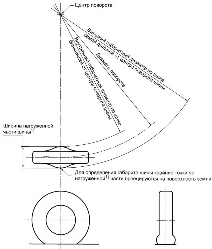
Рисунок 2 — Габаритные диаметры по шинам
