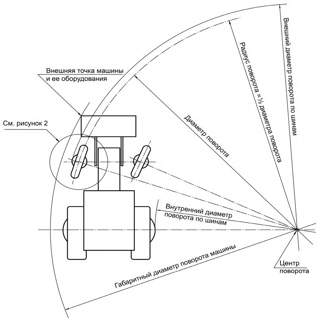
б) другие колесные машины
