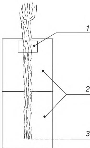
1 — взвешенная стеклянная пластина; 2 — бархатные доски; 3 — выровненный конец
