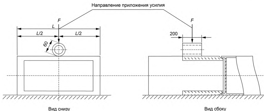
Рисунок 109 — Типовая испытательная установка для механических испытаний основания
