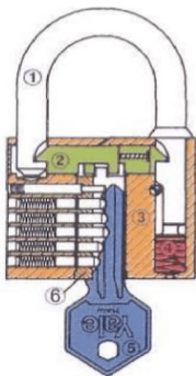
Устройство навесного замка с ЦМС с дужкой
