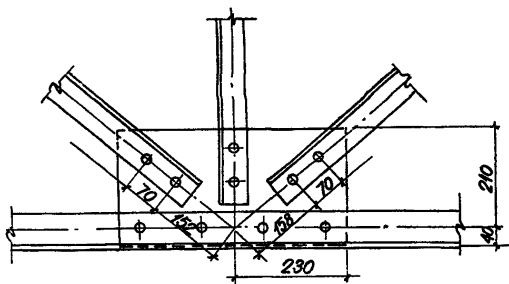
Рис. 25. Промежуточный узел нижнего пояса клепаной стропильной фермы
