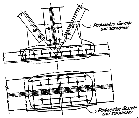
Рис. 28. Примеры решения стыков поясов клепаных ферм: а) стык верхнего пояса; б) стык нижнего пояса
